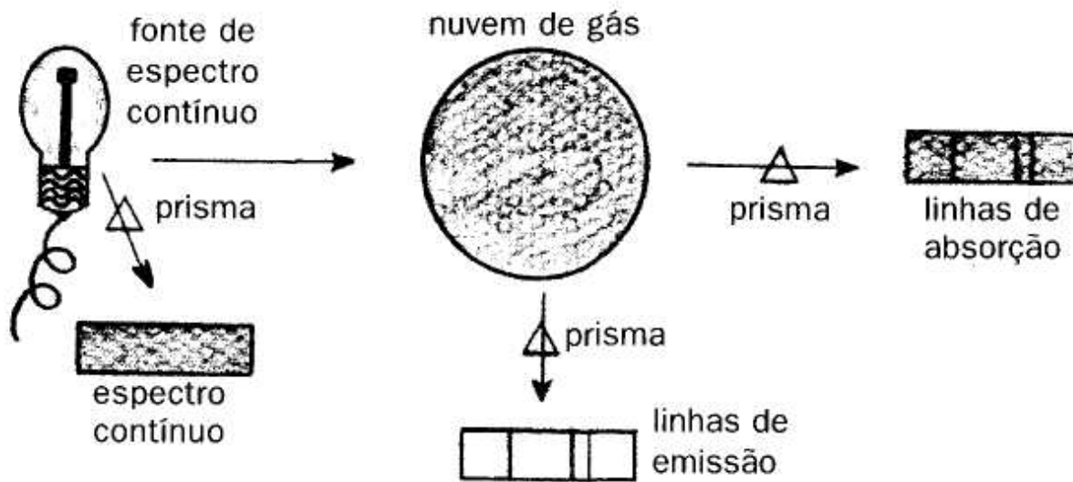
FIGURA 6.2: Espectros de emissão e absorção: uma nuvem de gás produz um espectro de emissão com algumas linhas brilhantes características (centro). Quando a mesma nuvem está
