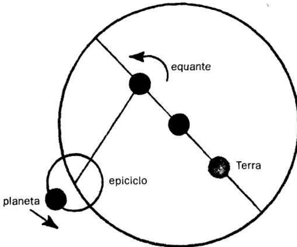
FIGURA 2.8: Diagrama mostrando o equante de Ptolomeu.
