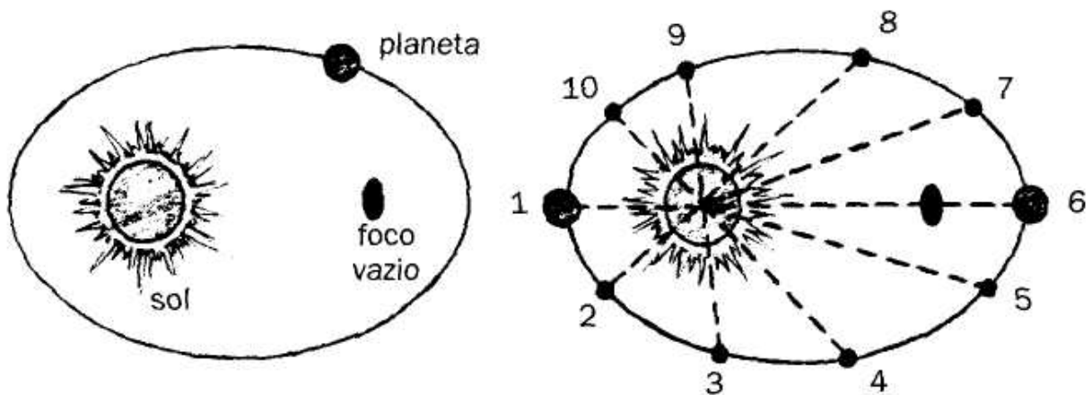
FIGURA 3.4: As duas primeiras leis de Kepler do
