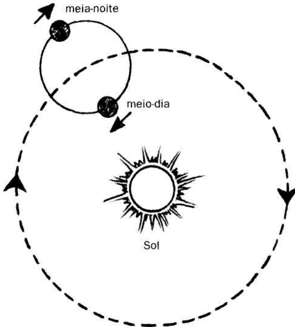
FIGURA 4.1: A teoria das marés de Galileu. A rotação da Terra em torno de seu eixo é representada esquematicamente, à meia-noite e ao meio-dia. Terra pode ser decomposto em duas partes, sua órbita em torno do Sol e sua rotação em torno de seu eixo. De acordo com Galileu, esses dois movimentos eram responsáveis pelo movimento dos oceanos, que causa as marés. Esse é basicamente seu argumento: considere uma cidade situada perto do oceano, como o Rio de Janeiro. Conforme indicado na figura 4.1, à meia-noite ambos os movimentos apontam na mesma direção, fazendo com que a terra firme "avance" para a frente mais rapidamente do que as águas dos oceanos. (Pense numa banheira com água sendo empurrada para a
