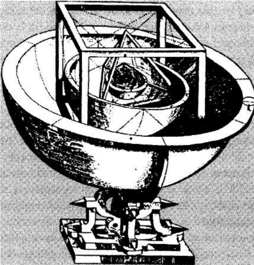
FIGURA 3.2: O Universo geométrico de Kepler.
