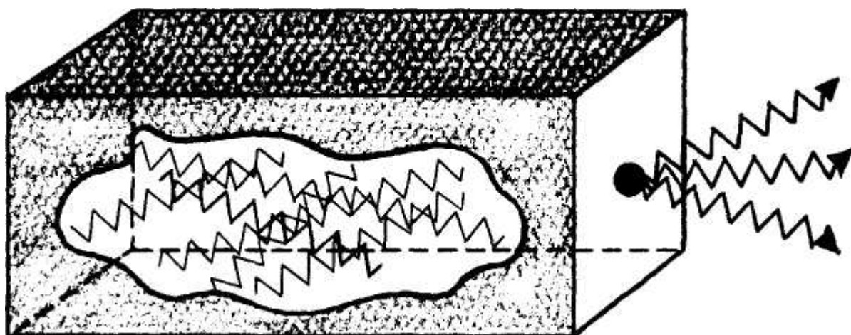
FIGURA 8.1: Um forno é aquecido a uma temperatura T . A radiação de corpo negro escapa através de um pequeno orifício numa das
