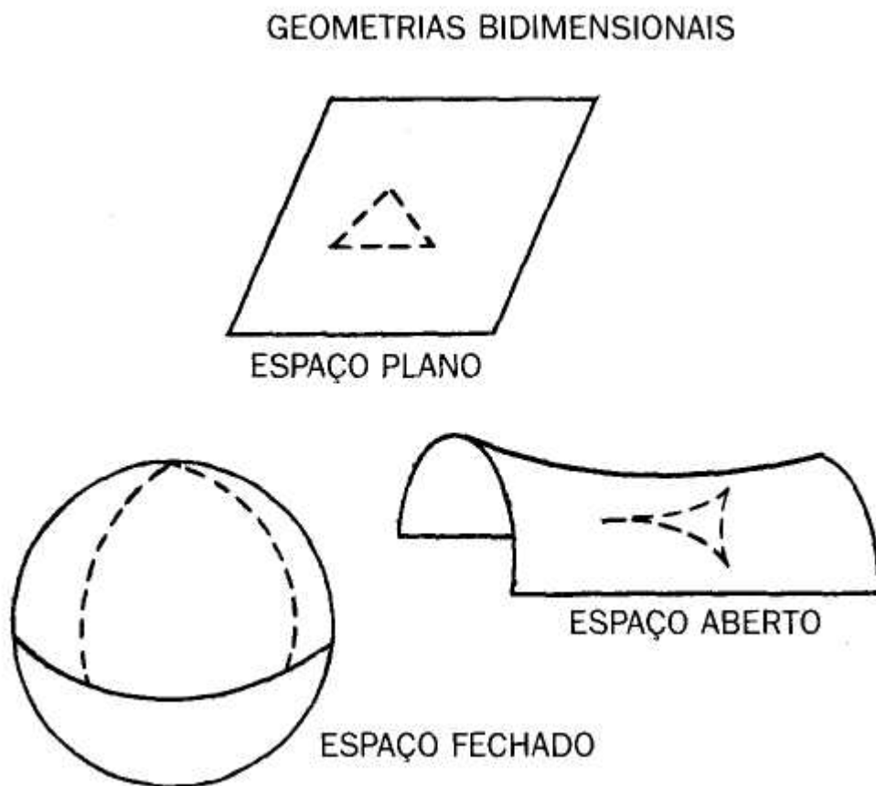
FIGURA 9.3: Geometrias não euclidianas bidimensionais: (no alto) Geometria plana com triângulo; (embaixo, à esquerda) Geometria fechada (curvatura positiva) com triângulo. A soma dos ângulos
