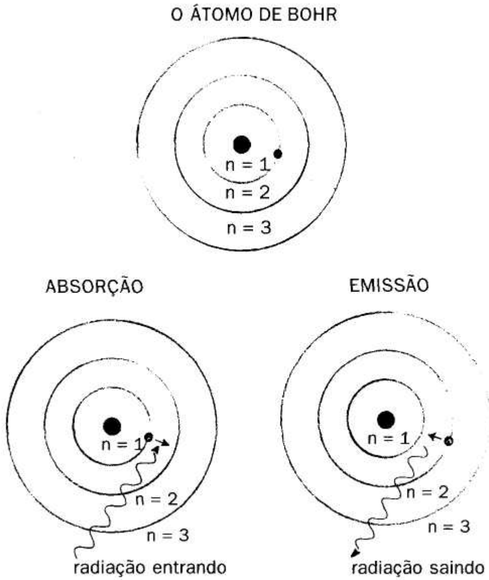
FIGURA 8.4: O modelo atômico de Bohr: os elétrons movem-se em torno do núcleo em órbitas circulares discretas. Ao absorver um fóton, o elétron poderá “saltar” para uma órbita mais elevada. Ao “relaxar”, passando de uma órbita mais elevada para uma mais próxima do estado fundamental, o elétron emitirá um fóton. Em ambos os casos, a energia do fóton é idêntica à diferença de energia entre as duas órbitas.
