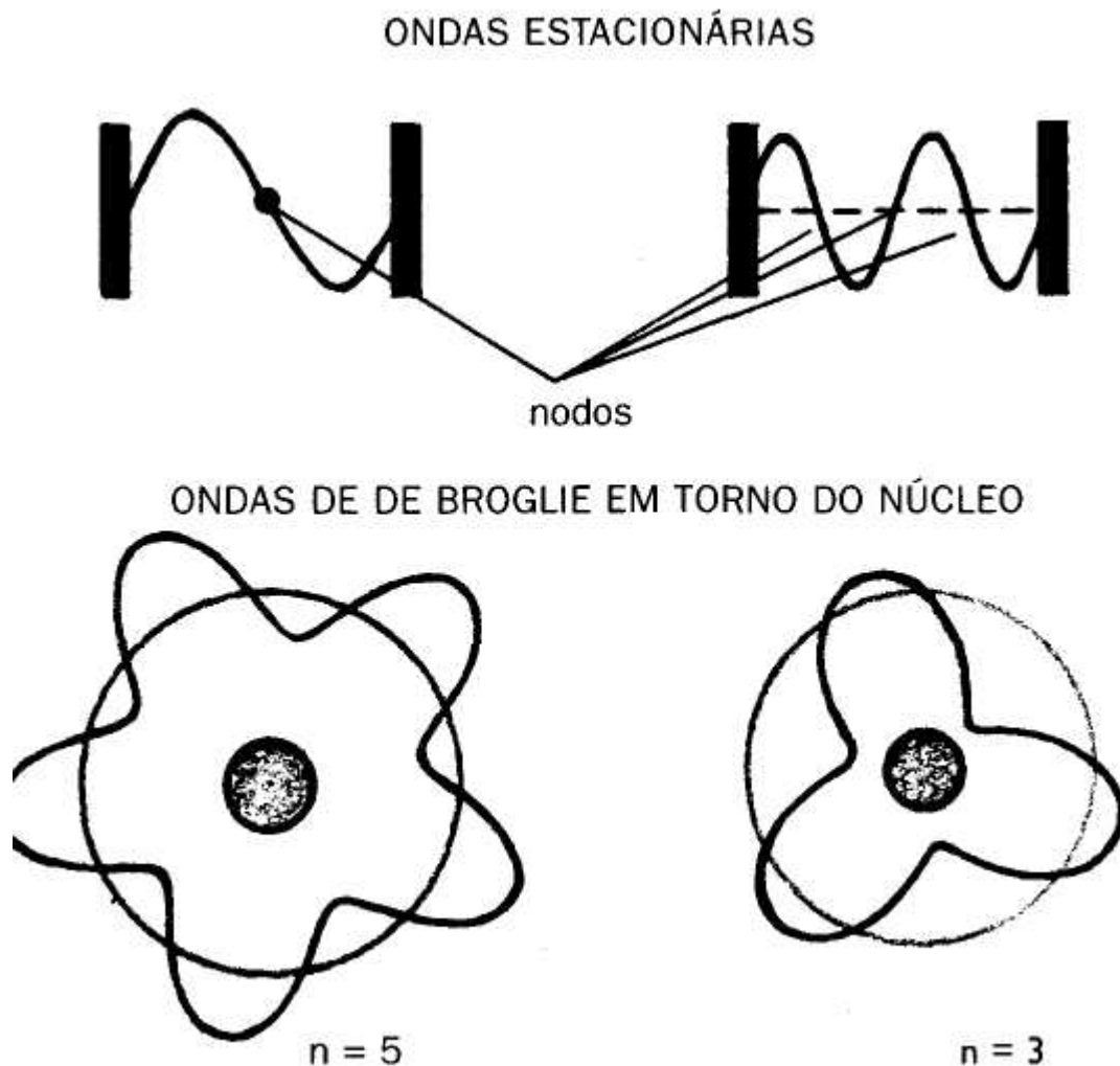
FIGURA 8.5: Ondas estacionárias são caracterizadas pelo seu número inteiro de nodos. De Broglie imaginou o elétron como sendo uma onda estacionária ao redor do núcleo. A energia da órbita eletrônica tem uma correspondência unívoca com o número de nodos da onda estacionária: quanto maior o número de nodos, maior a distância entre a órbita e o núcleo.
