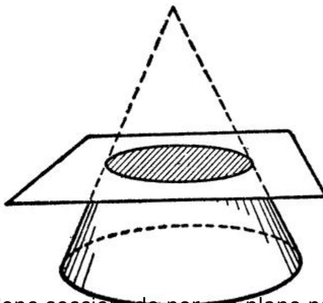
Figura 16: Cone seccionado por um plano paralelo à sua base.
