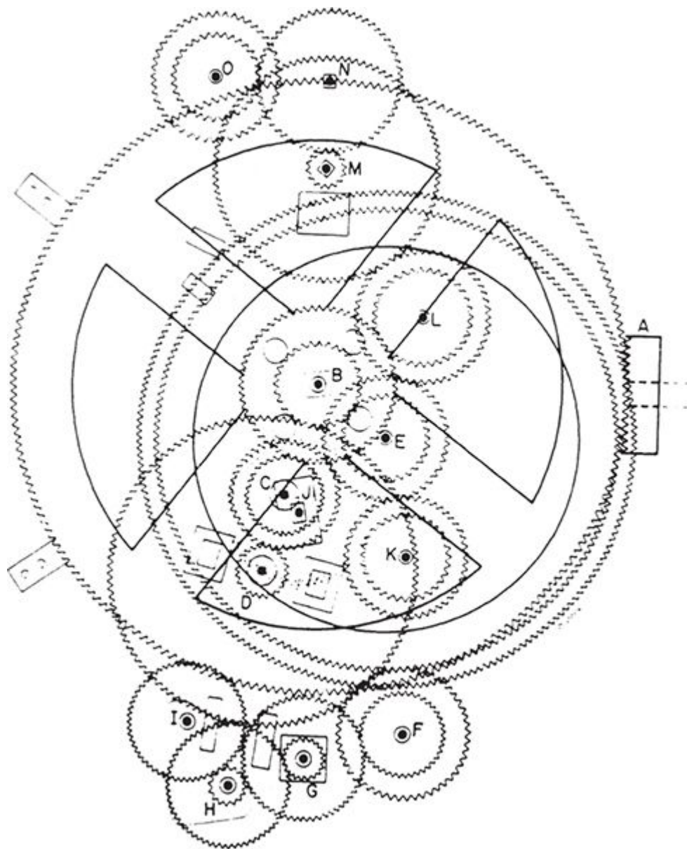
FIGURA 8. Engrenagem do mecanismo de Anticítera, antigo calculador planetário grego.
