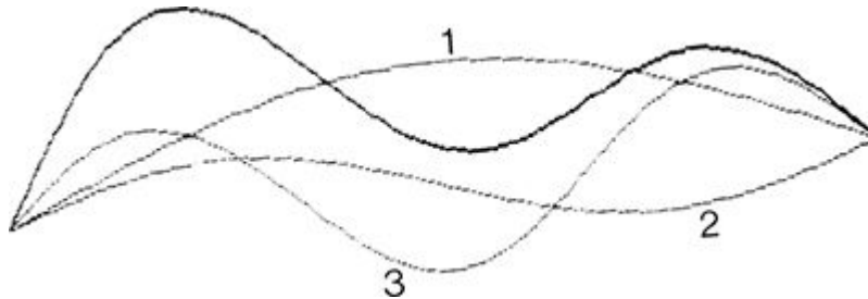
FIGURA 13. Vibração de uma corda de violino: senoide fundamental (1) e seus segundo e terceiro harmônicos (2, 3), superpostos para criar uma onda mais complexa (linha cheia).
