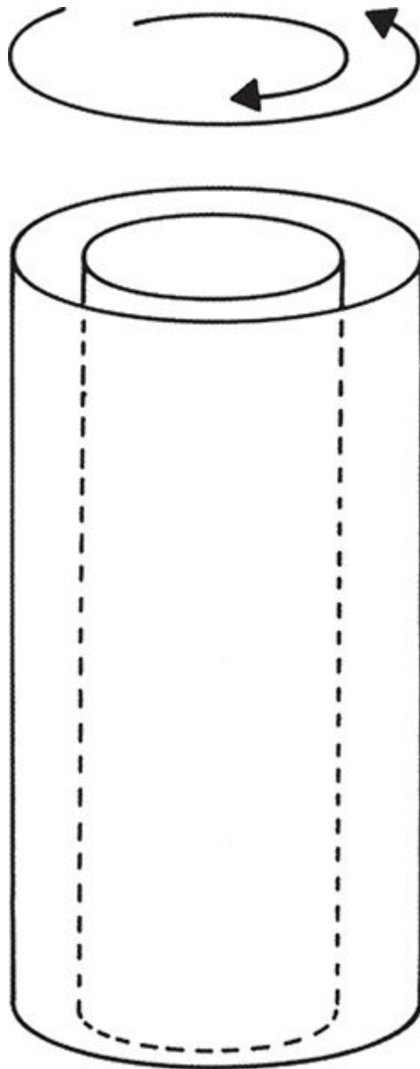
FIGURA 72. Aparelho para o experimento de Taylor-Couette (esquema). O espaço entre dois cilindros é preenchido com fluido, e os cilindros são girados. A distância entre os cilindros foi exagerada aqui, para efeito de maior clareza: em geral é de 10 a 20% do raio do cilindro externo.
