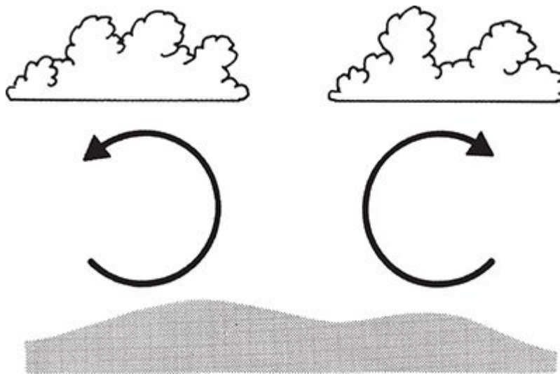
FIGURA 53. Células de convecção, causadas pela subida do ar quente.
