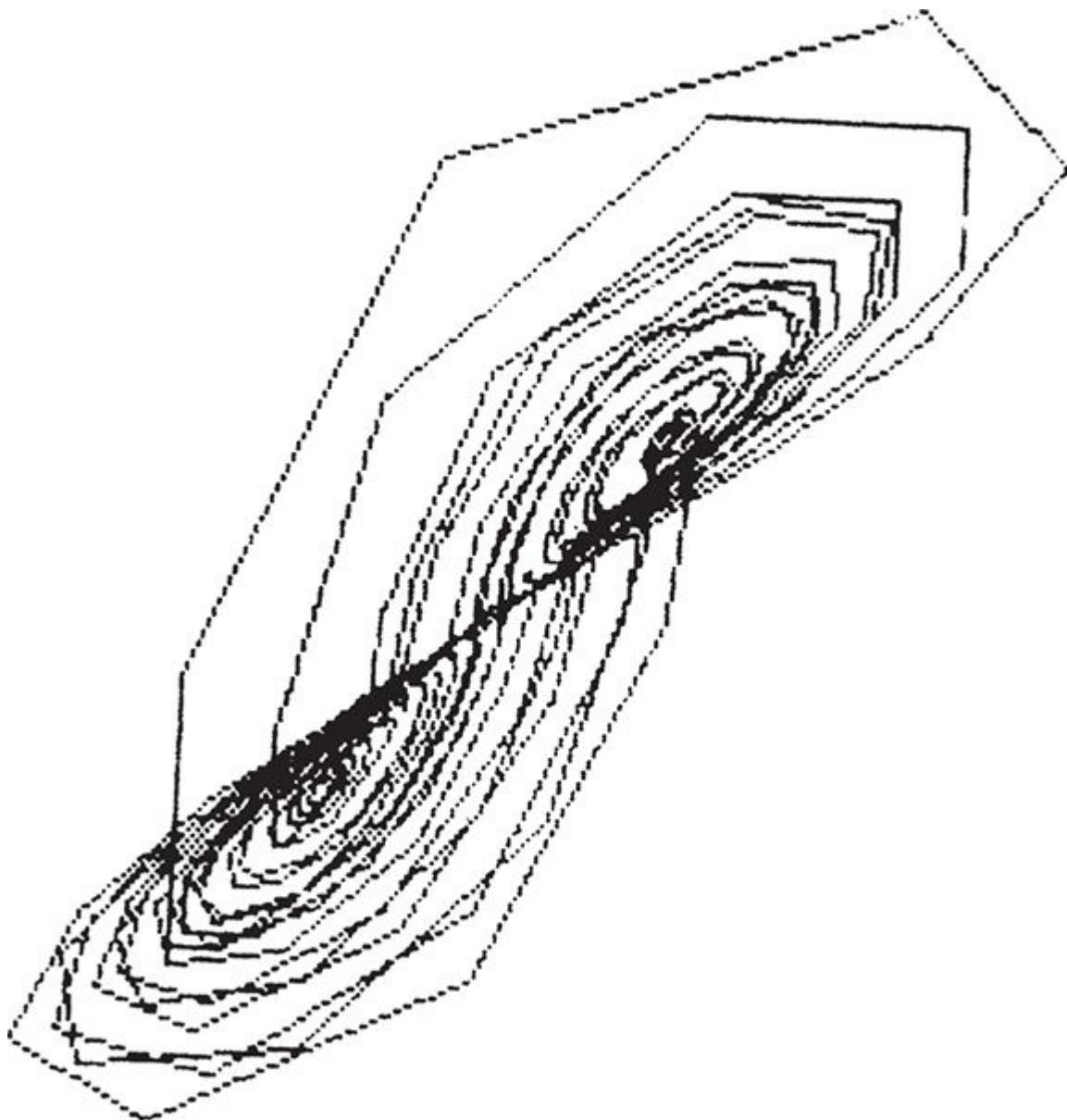
FIGURA 77. Reconstrução de um atrator estranho (aqui o atrator de Lorenz) pelo método de Packard-Takens (compare com a figura 54).
