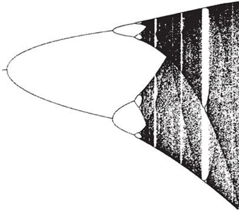
FIGURA 65. Diagrama das bifurcações para o mapeamento logístico. A constante k aumenta de 2 para 4 na horizontal. A coordenada vertical é o estado x . Observe a figueira de duplicações de períodos, seguida pelo crescimento de faixas caóticas. (Reproduzido com a permissão de John Wiley & Sons Ltd.)
