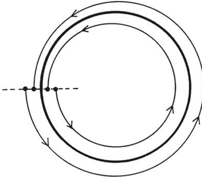
FIGURA 45. A seção de Poincaré (linha pontilhada) através de um ciclo-limite (linha cheia): pontos iniciais da seção de Poincaré se contraem em direção ao ponto que representa o ciclo-limite em seu primeiro retorno.
