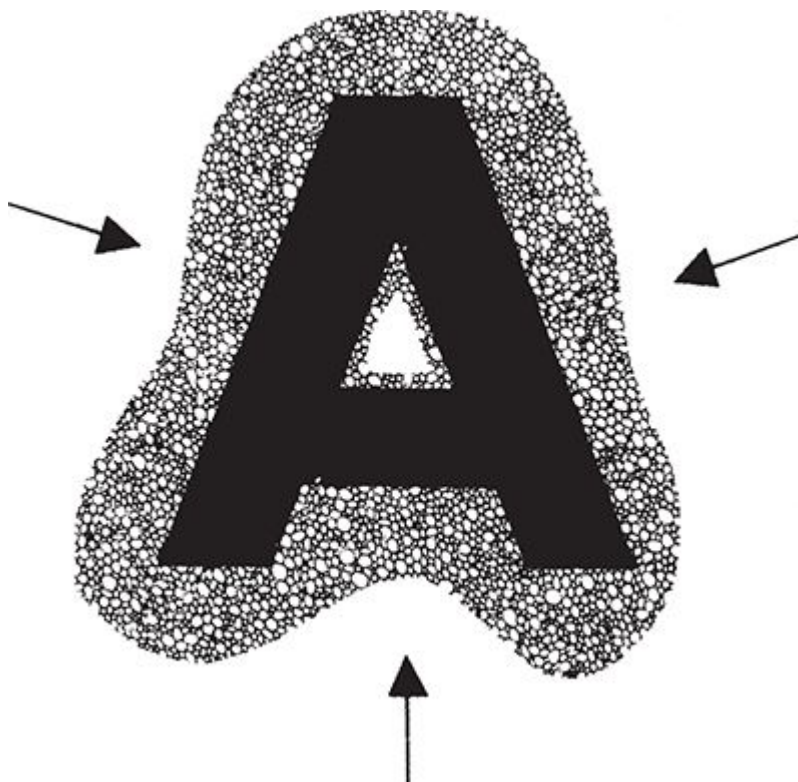
FIGURA 43. Representação esquemática de um atrator genérico, mostrado aqui como na forma de um A negro: regiões próximas (sombreadas) se contraem em direção ao atrator à medida que o tempo passa.
