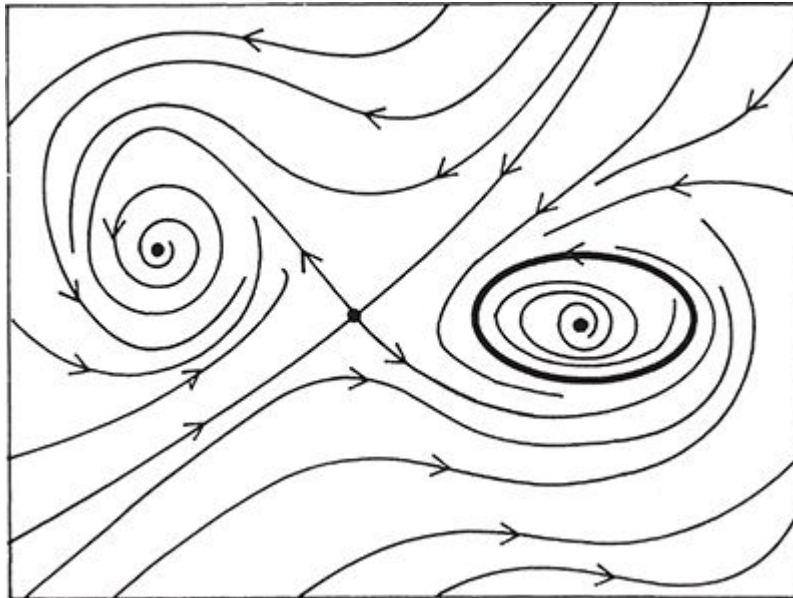
FIGURA 36. Retrato de fase de um fluxo no plano, mostrando (da esquerda para a direita) um sumidouro, uma sela, um ciclo-limite e uma fonte.
