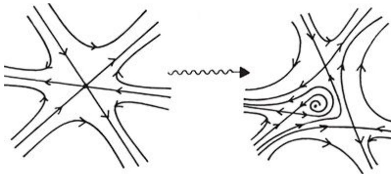
FIGURA 42. Instabilidade estrutural: uma sela com três separatrizes se desagrega sob pequenas perturbações, formando três selas separadas e um sumidouro.
