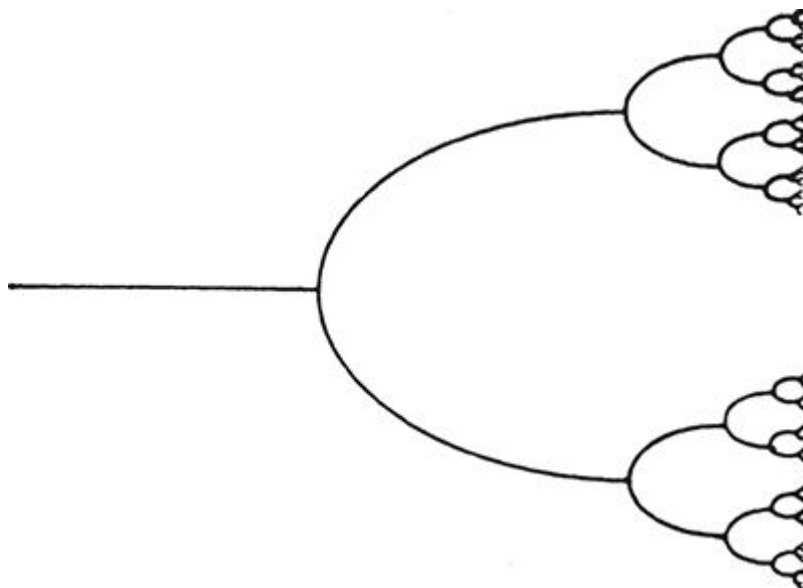
FIGURA 66. Visão esquemática da figueira: ramificação regular, repetitiva, com ramos infinitamente numerosos ocorrendo num espaço finito.
