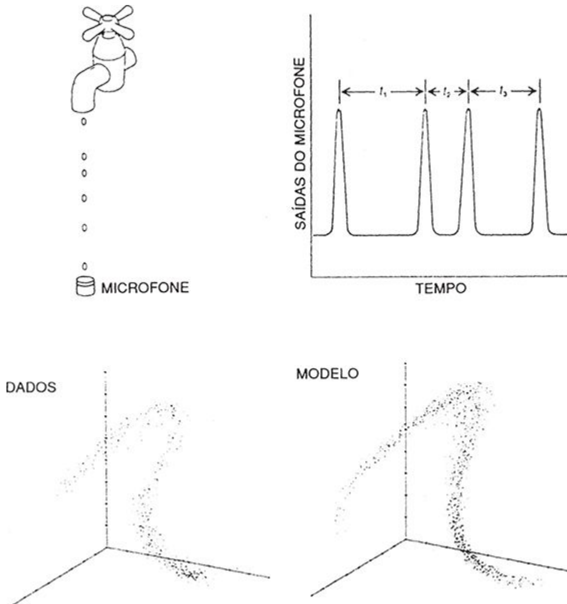
FIGURA 80. O experimento da torneira que pinga: (no alto, à esquerda) aparelhagem, (no alto, à direita) parte de uma série temporal, (embaixo, à esquerda) uma representação tridimensional dos dados observados, (embaixo, à direita) um modelo matemático simples.
