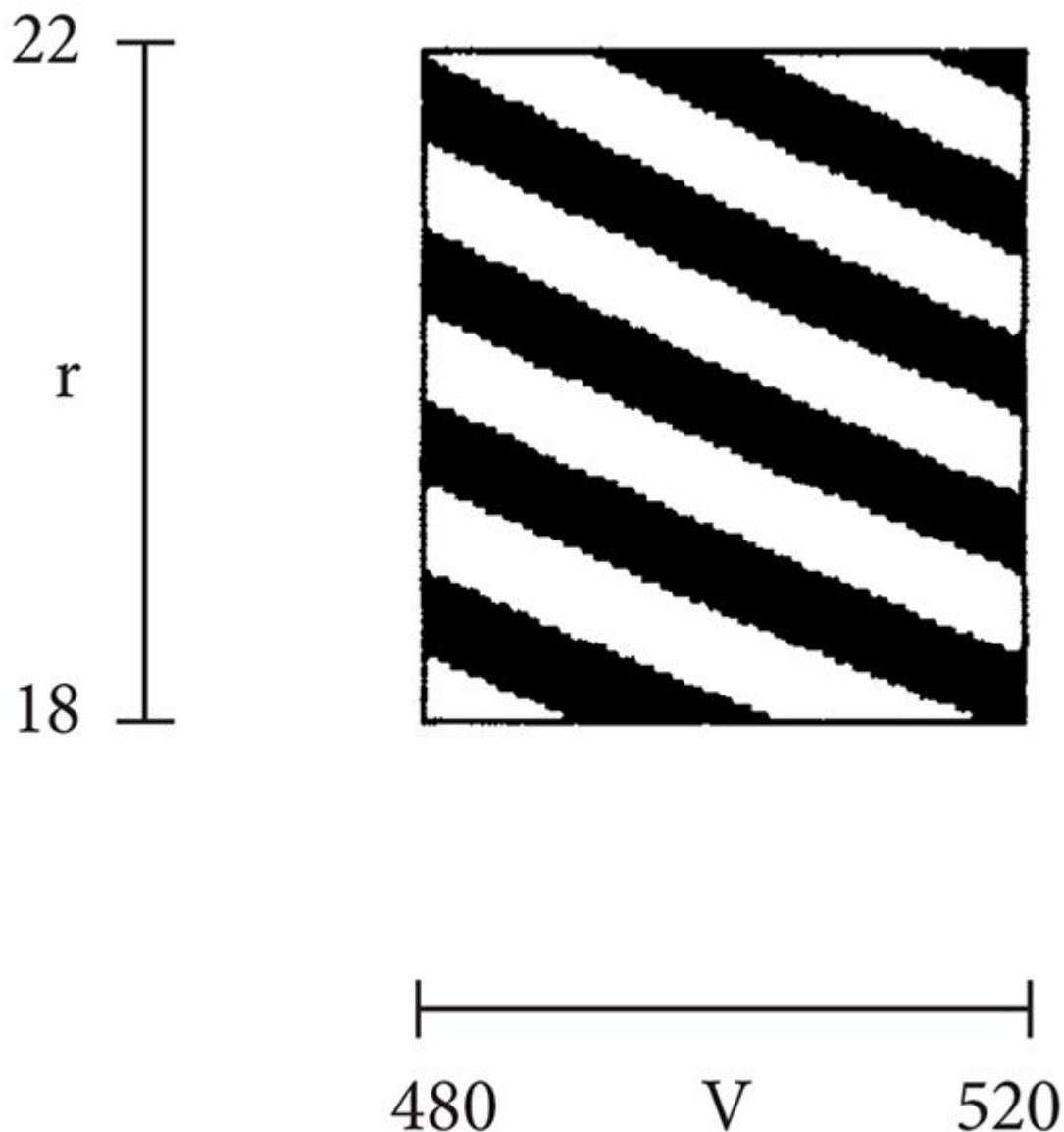
FIGURA 124. Condições iniciais para uma moeda girando, com listras que correspondem a seu destino final. Preto = coroa; branco = cara.
