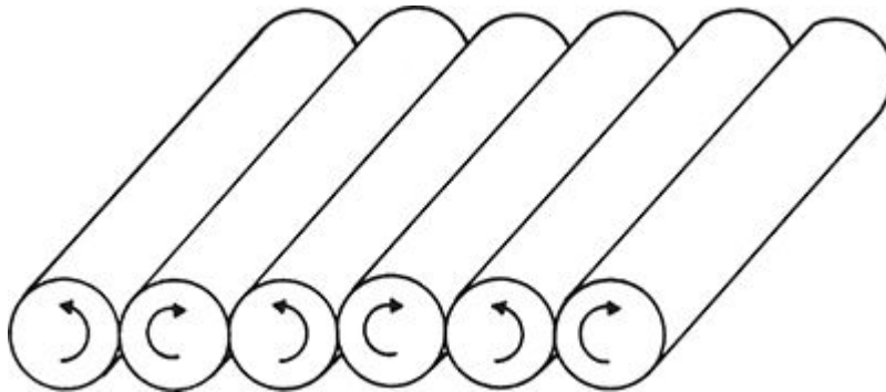
FIGURA 86. Rolos paralelos na convecção em fluidos: rolos vizinhos giram em direções opostas.
