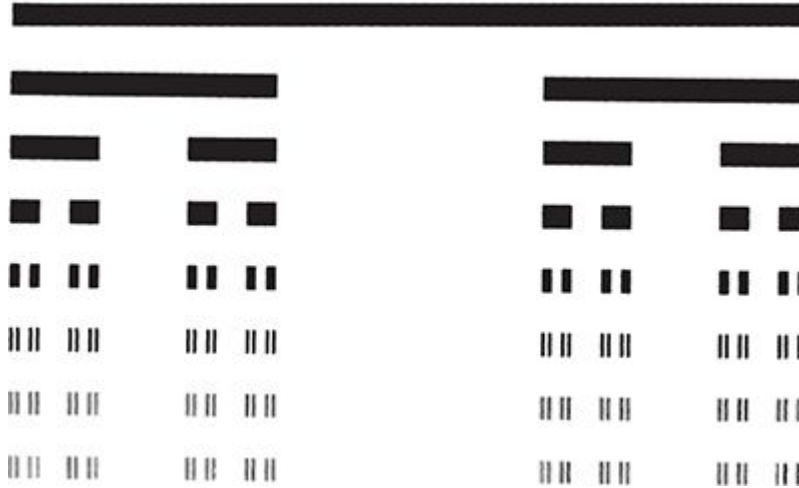
FIGURA 49. A construção do conjunto de Cantor pela supressão repetida das terças partes intermediárias. A dimensão vertical foi exagerada para fins de clareza: idealmente, a linha não tem largura.
