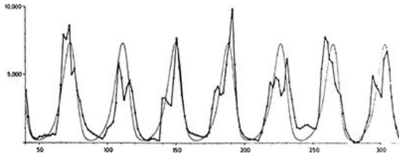
FIGURA 115. Modelo da oscilação básica nos dados sobre as moscas-varejeiras, incorporando efeitos de retardamento.
