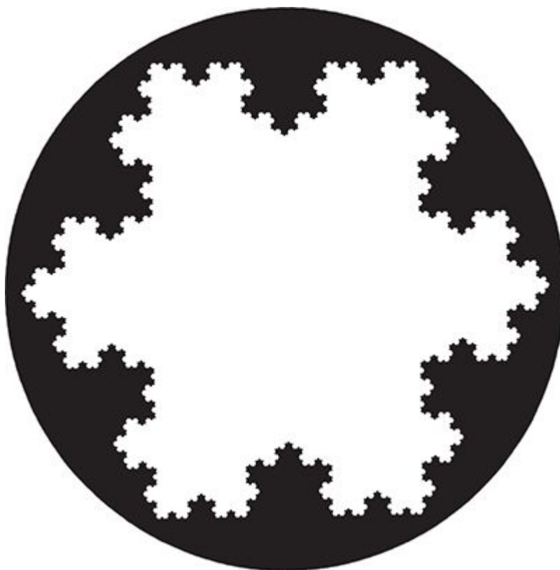
FIGURA 89. A curva do floco de neve, um fractal matemático.
