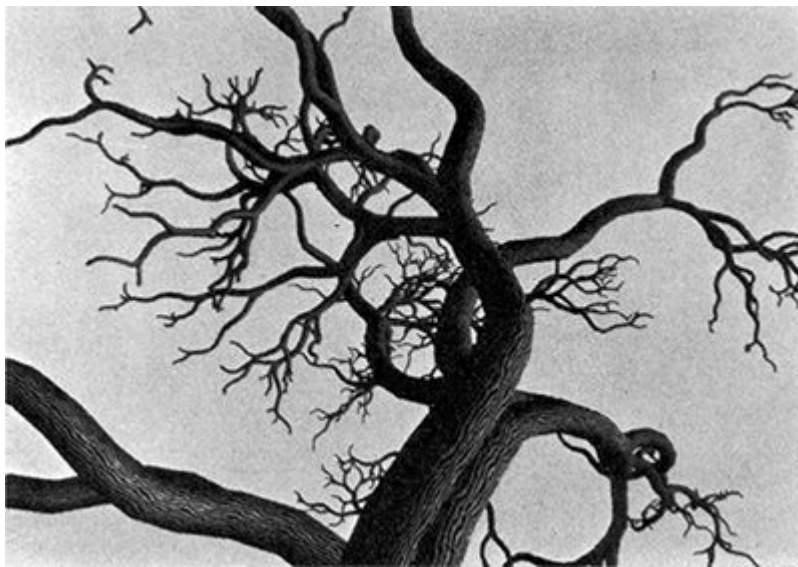
FIGURA 97. Simulação fractal de uma árvore. (New York Institute of Technology [Peter Oppenheimer].)
