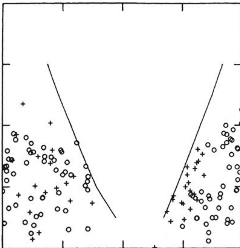
FIGURA 112. Fronteiras da zona caótica 3:1: teoria e observação. Na teoria, a região entre as duas linhas não devia conter asteroide algum. Os pontos e as cruces, que representam valores observados, confirmam essa previsão.
