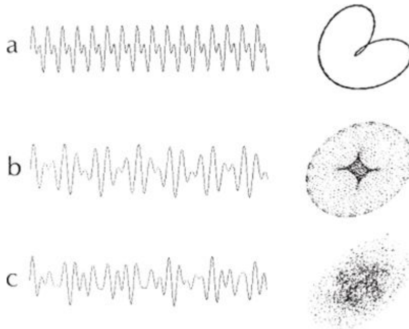
FIGURA 76. Experimentos de computador na reconstrução de atratores pelo método de Packard-Takens, numa representação bidimensional: (a) a série temporal periódica \sin t + \sin 2t gera uma volta fechada; (b) a série temporal com duas frequências \sin t + \sin \sqrt{2}t dá (uma projeção de) um toro; (c) a série temporal com três frequências \sin t + \sin \sqrt{2}t + \sin \sqrt{3}t não tem estrutura clara numa representação bidimensional. Uma terceira coordenada precisa ser representada para revelar sua natureza quase-periódica.
