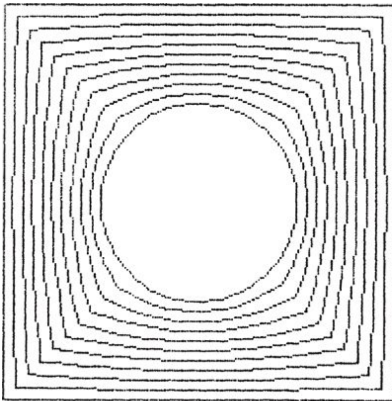
FIGURA 22. Para um topologista, quadrados e círculos são a mesma coisa, uma vez que um pode ser continuamente deformado até se converter no outro.
