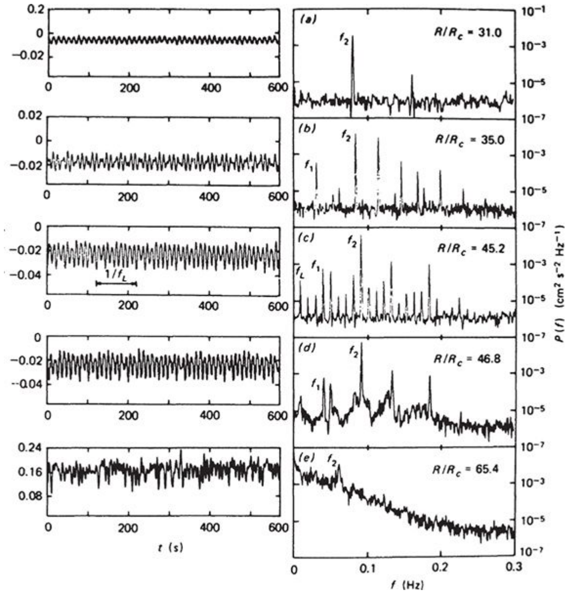
FIGURA 74. Séries temporais de observações num experimento com convecção e a sequência correspondente de espectros de potência, que mostra como mudam as intensidades das frequências componentes. Os picos indicam frequências bem definidas num movimento periódico ou quase-periódico; bandas largas indicam caos.
