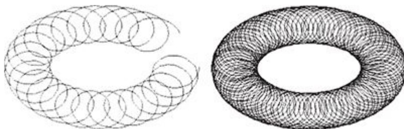
FIGURA 41. Topologicamente, movimentos quase-periódicos ocorrem num toro: (à esquerda) combinação de movimentos em pequenos e grandes círculos; (à direita) o toro resultante.
