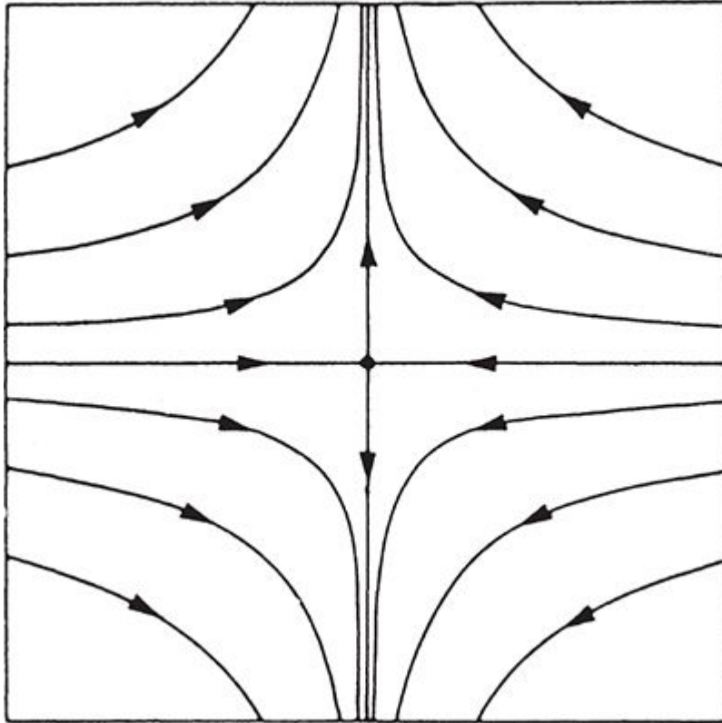
FIGURA 39. Uma sela: as linhas que se cruzam no centro são suas separatrizes.
