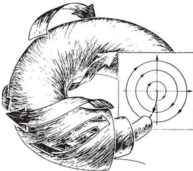
FIGURA 107. A figura clássica de uma seção de Poincaré nas proximidades de uma trajetória periódica. Cada círculo representa um movimento quase-periódico com dois períodos diferentes.
