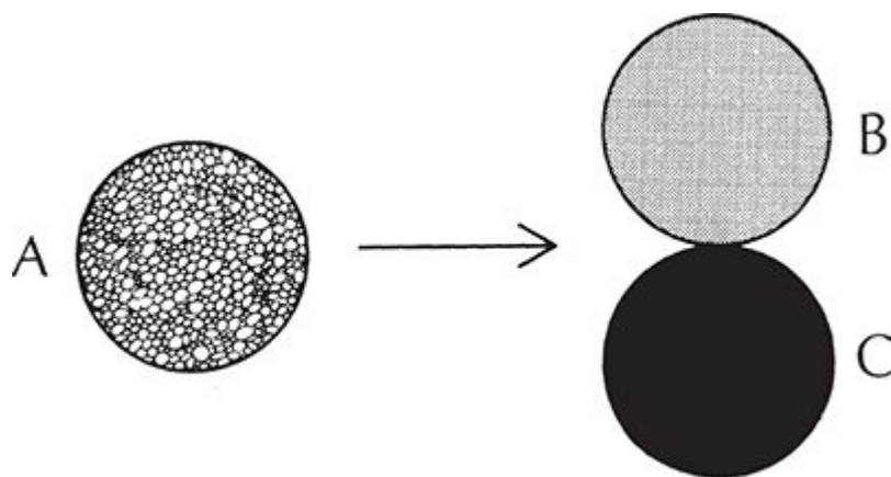
FIGURA 14. Para onde irão elas? Segundo as leis do movimento de Newton, e pressupondo que são esferas perfeitamente elásticas, os resultados dependem do que A atingirá primeiro: B ou C. Caso se choque com ambas ao mesmo tempo, as leis de Newton não especificam o que acontece.
