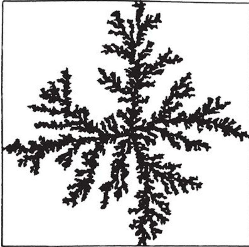
FIGURA 92. Aglomerado de partículas por DLA, desenvolvido num computador. (Reprodução autorizada de Nature , vol. 322, p.791, © Macmillan Magazines Ltd.)
