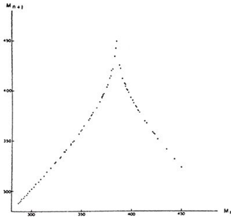
FIGURA 56. Ordem no caos. Representando-se o tamanho de uma oscilação comparado ao da oscilação prévia, obtém-se uma curva precisa. (American Meteorological Society, Journal of the Atmospheric Sciences , vol. 20 [Edward N. Lorenz].)
