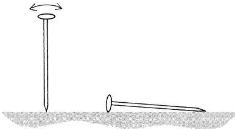
FIGURA 21. Um prego equilibrado na ponta é instável e na prática cairá. Deitado de lado, é estável.
