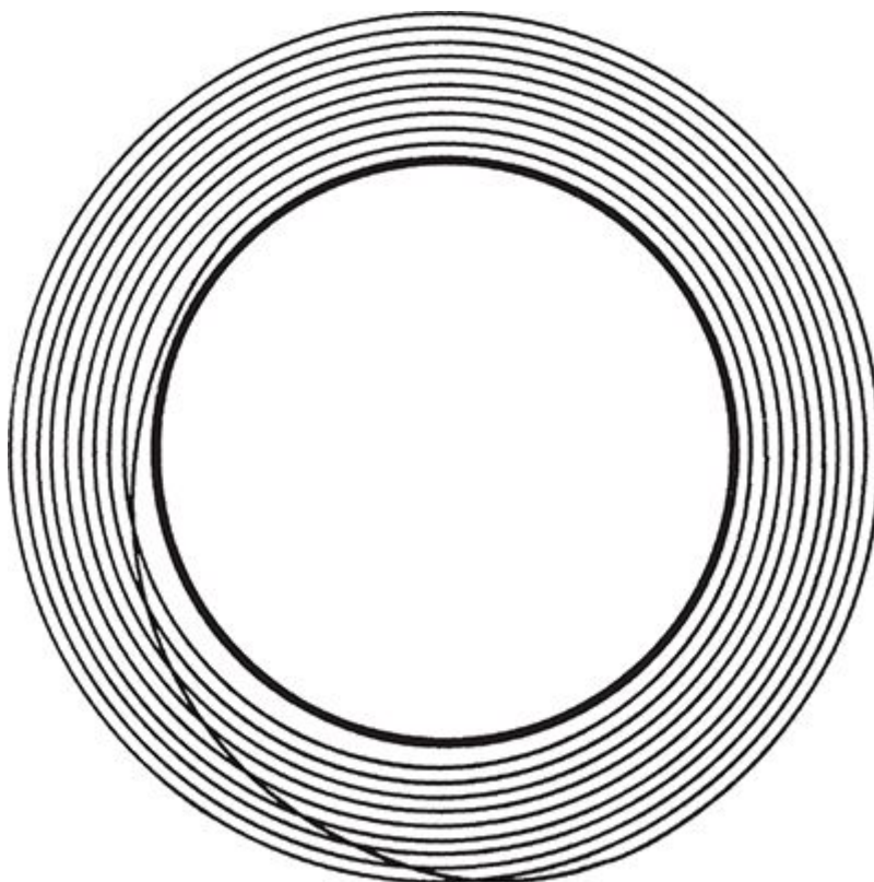
FIGURA 44. Um círculo esticado e enrolado dez vezes em torno de si mesmo (representação esquemática).
