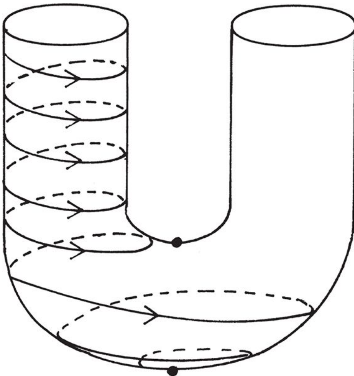
FIGURA 33. O amortecimento dissipa a energia: um pêndulo amortecido desce pela espiral dos níveis de energia.
