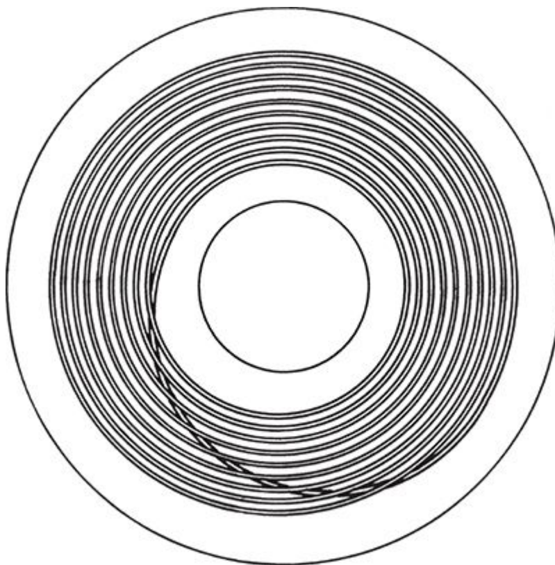
FIGURA 48. O enrolamento por dez vezes aplicado a um toro sólido para evitar autointerseções. Como o toro é tridimensional, há espaço para que uma volta passe sob as outras sem tocá-las.
