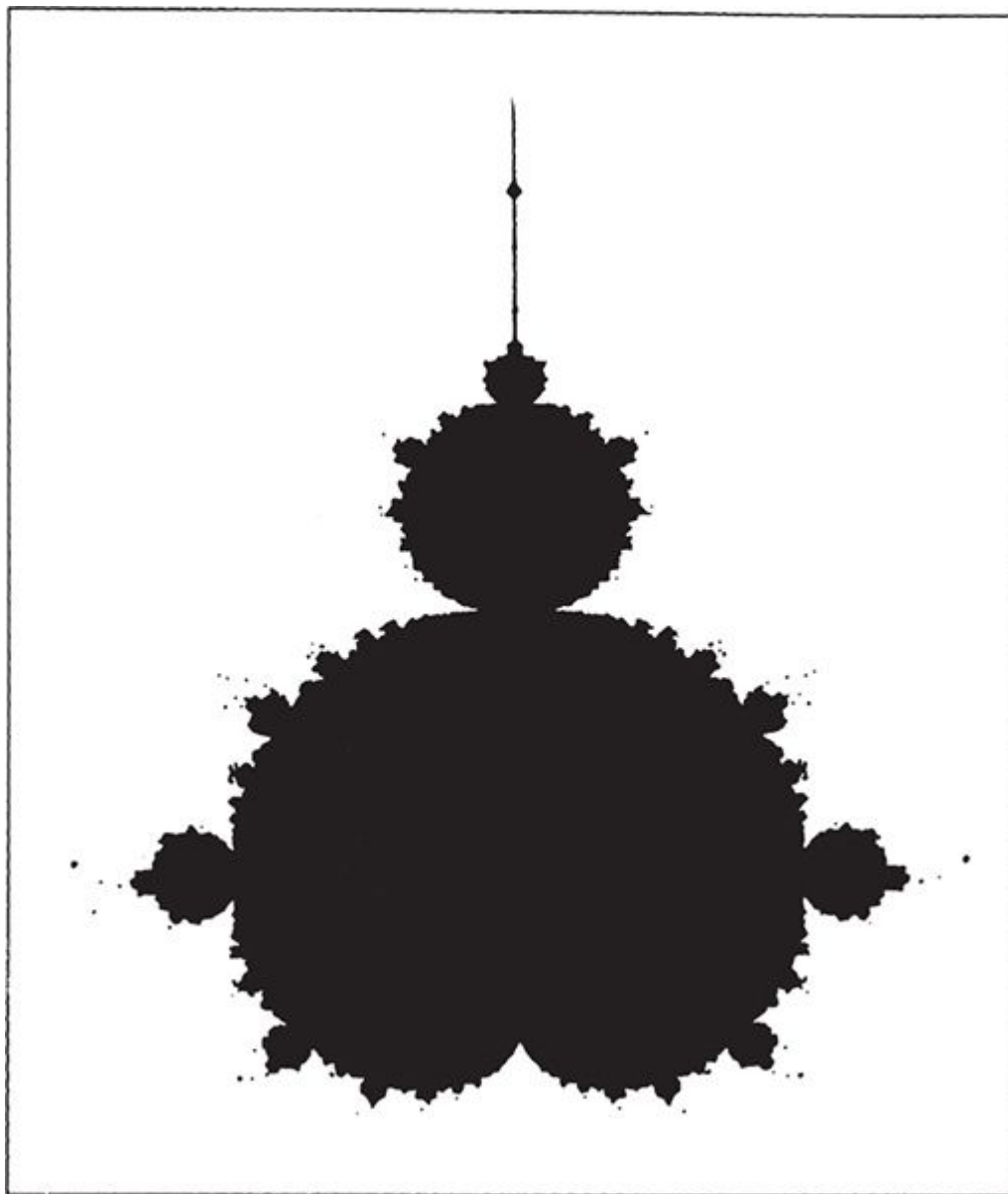
FIGURA 100. O conjunto de Mandelbrot ou o “boneco de pão de mel”. (Reprodução autorizada de H.-O. Peitgen e P.H. Richter: The Beauty of Fractals , 1986. © 1986 Springer-Verlag Berlin – Heidelberg.)
