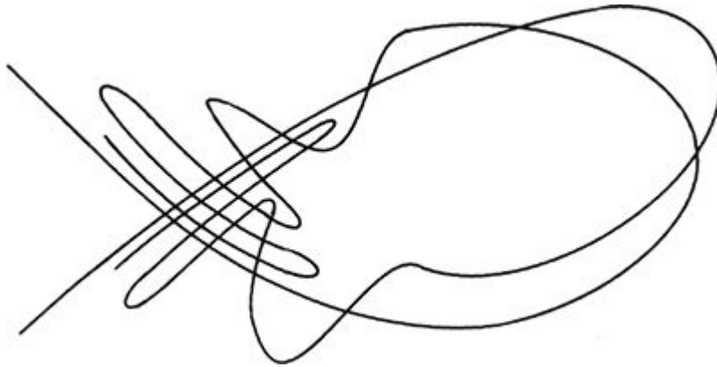
FIGURA 26. Pegadas do caos na poeira dos tempos... Emaranhados homoclínicos no problema dos três corpos. Poincaré ficou aterrorizado.
