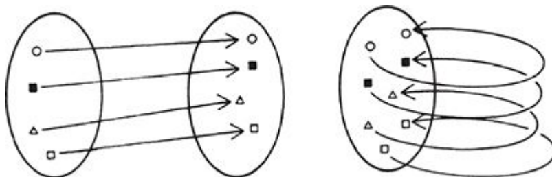
FIGURA 47. Suspensão: um truque matemático para transformar um mapeamento (à esquerda) num fluxo num espaço com uma dimensão a mais (à direita).
