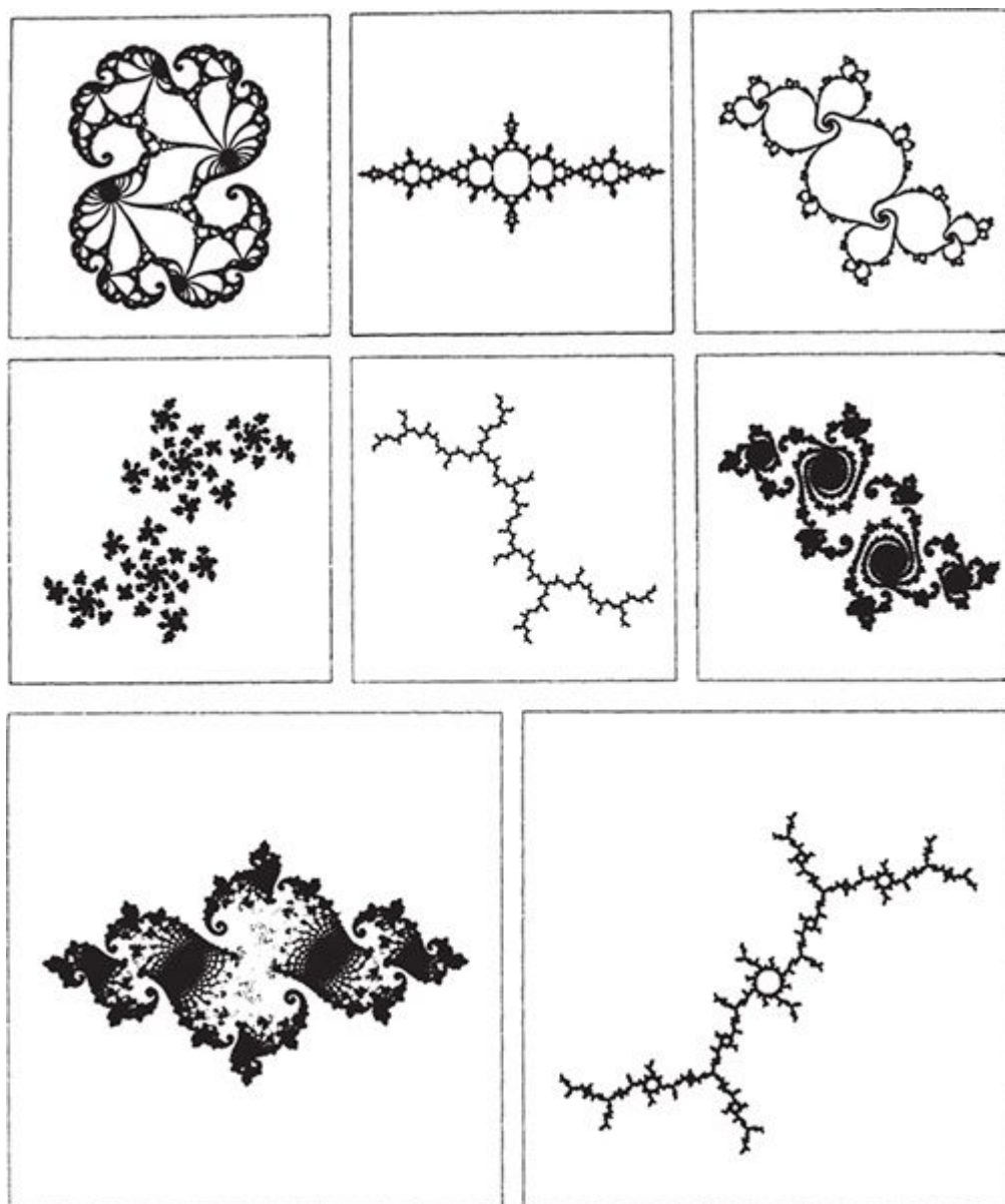
FIGURA 99. Conjuntos de Júlia: uma ideia simples conduz a uma intrincada beleza e a uma variedade inesgotável.
