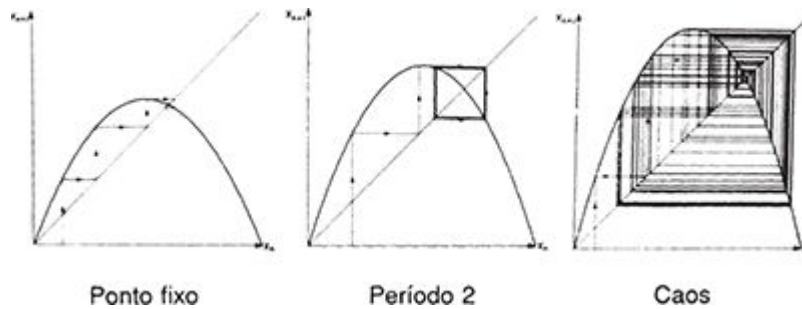
FIGURA 61. Iteração gráfica do mapeamento logístico feita com diagramas da teia de aranha (da esquerda para a direita): estado estacionário, ponto periódico, caos. (Reproduzido com a permissão de John Wiley & Sons Ltd.)
