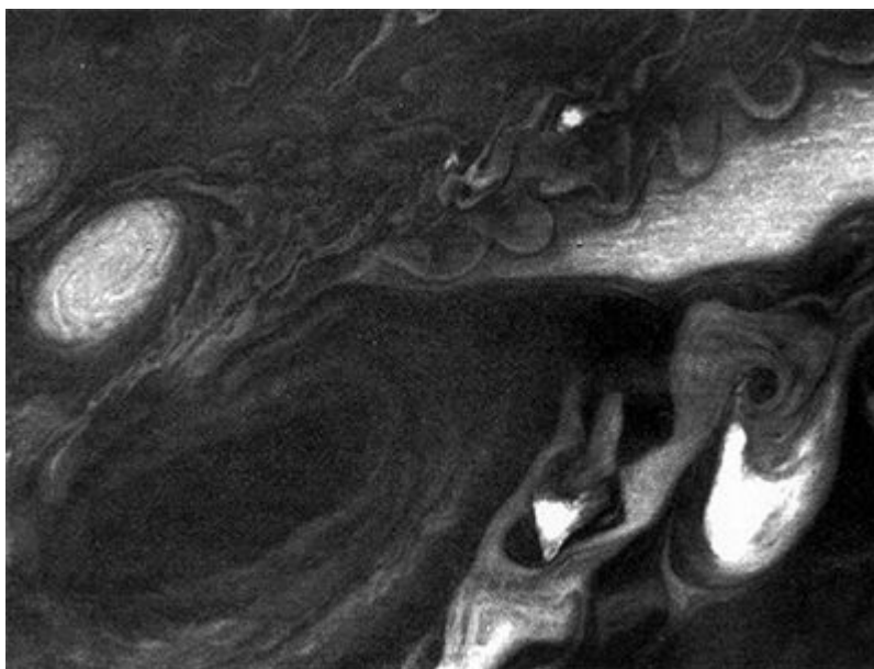
FIGURA 69. Turbulência na atmosfera de Júpiter, próximo da Grande Mancha Vermelha
