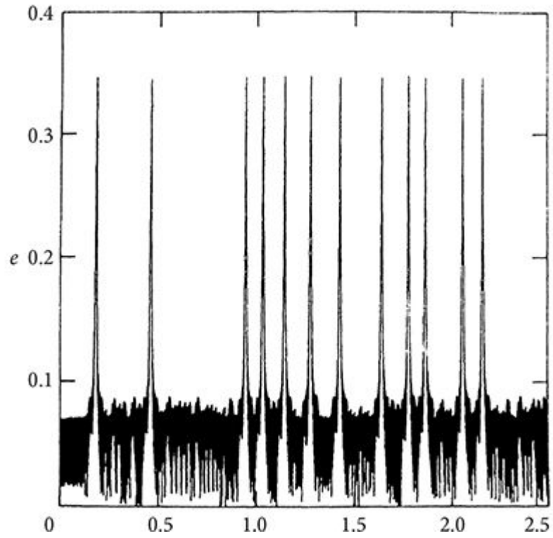
FIGURA 110. A excentricidade e da órbita de um asteroide em ressonância 3:1 com Júpiter. Os picos correspondem a mudanças repentinas e grandes na excentricidade. A escala de tempo horizontal t é em milhões de anos.
