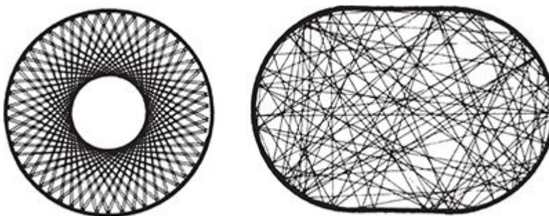
FIGURA 122. Bilhar clássico, uma chave para o caos quântico. Uma partícula ricocheteia nos limites de alguma região, como uma bola numa mesa de bilhar. Um anel circular (à esquerda) leva a comportamento regular. O estádio de Bunimovich (à direita) leva ao caos.
