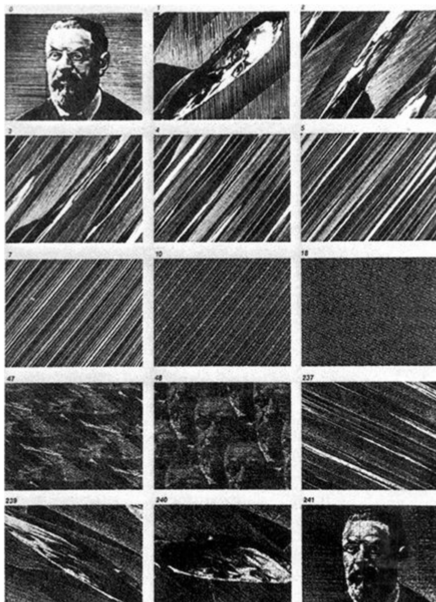
FIGURA 20. Retrato de Henri Poincaré, ilustrando sua descoberta da “recorrência de Poincaré”. Se uma transformação é aplicada repetidamente a um sistema matemático que não possa sair de uma região limitada, este deverá retornar um número infinito de vezes a estados próximos ao seu estado original.
