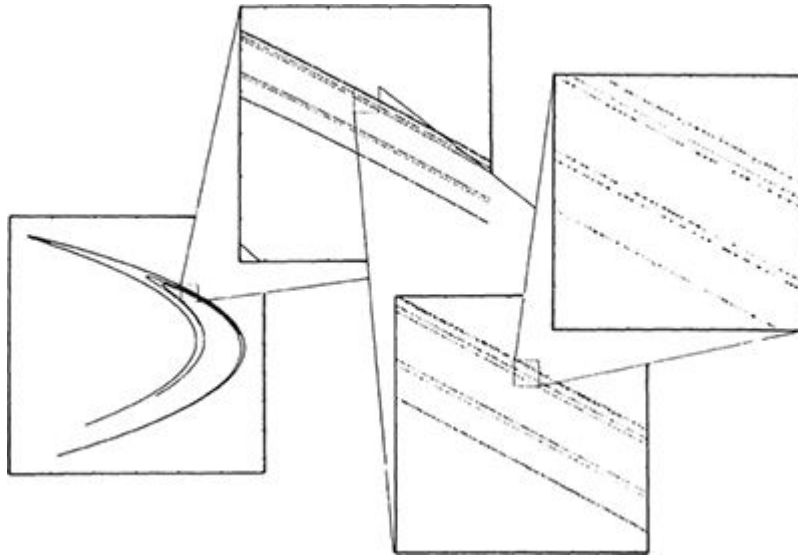
FIGURA 60. A estrutura em finas camadas do atrator de Hénon.
