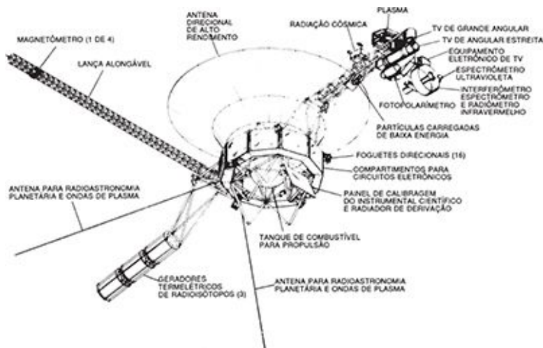
FIGURA 4. A nave espacial Voyager 1 .
