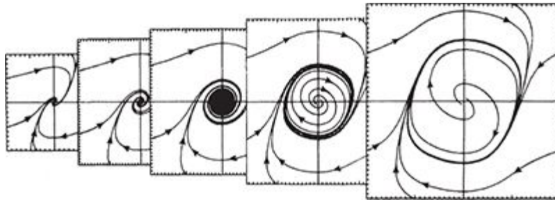
FIGURA 70. Surgimento de uma oscilação, ou como um estado estacionário se torna periódico. O mecanismo é chamado de bifurcação de Hopf: um sumidouro perde a estabilidade e se torna uma fonte, gerando um ciclo-limite. (Reproduzido com a permissão de John Wiley & Sons Ltd.)
