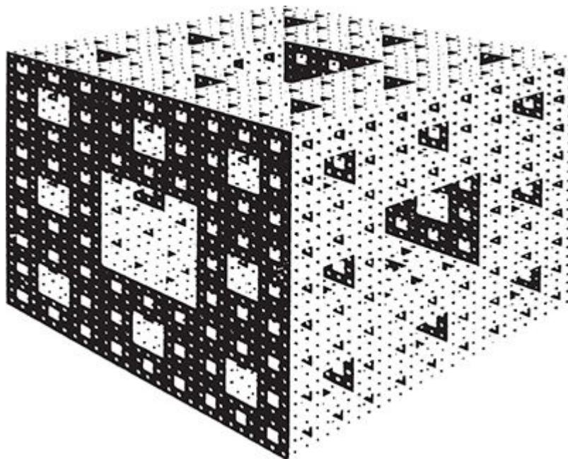
FIGURA 90. A esponja de Menger, um fractal de dimensão \log 20/\log 3 = 2,7268 .
