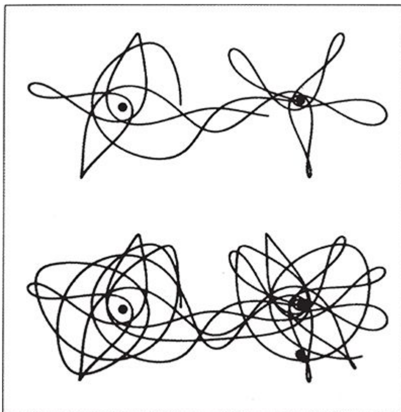
FIGURA 23. As complexidades do movimento de três corpos: aqui uma partícula de poeira se move na órbita de dois planetas fixos de massas iguais.
