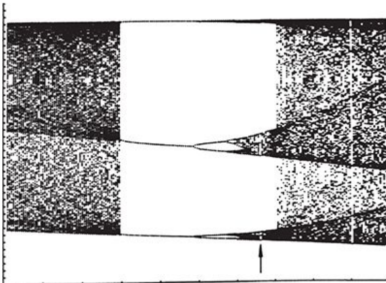
FIGURA 67. Detalhe da figura 65, no interior de uma janela periódica: a estrutura inteira se repete em miniatura. E há janelas dentro de janelas (indicadas pela seta)... (Reproduzido com a permissão de John Wiley & Sons Ltd.)
