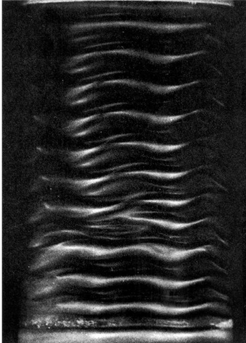
FIGURA 73. Vórtices ondulados no experimento de Taylor-Couette. Observe o deslocamento, a dois terços do caminho, de cima para baixo, onde o número de ondas no processo está se modificando.
