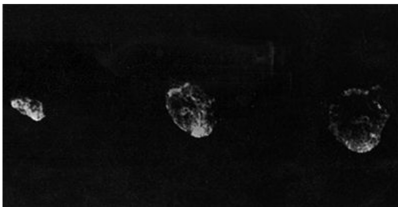
FIGURA 104. Três imagens da Voyage mostrando Hipérion, o satélite indisciplinado de Saturno.
