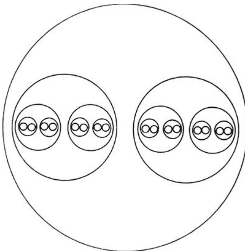
FIGURA 50. O queijo de Cantor: construção alternativa de um equivalente topológico do conjunto de Cantor, usando pares de círculos.
