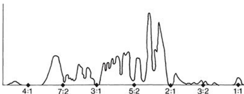
FIGURA 109. Os asteroides formam aglomerados a algumas distâncias do Sol e deixam lacunas a outras. Ao que parece, isso é provocado por ressonâncias com Júpiter. O gráfico representa a proporção de asteroides versus a razão entre o período de Júpiter e o período dos asteroides.
