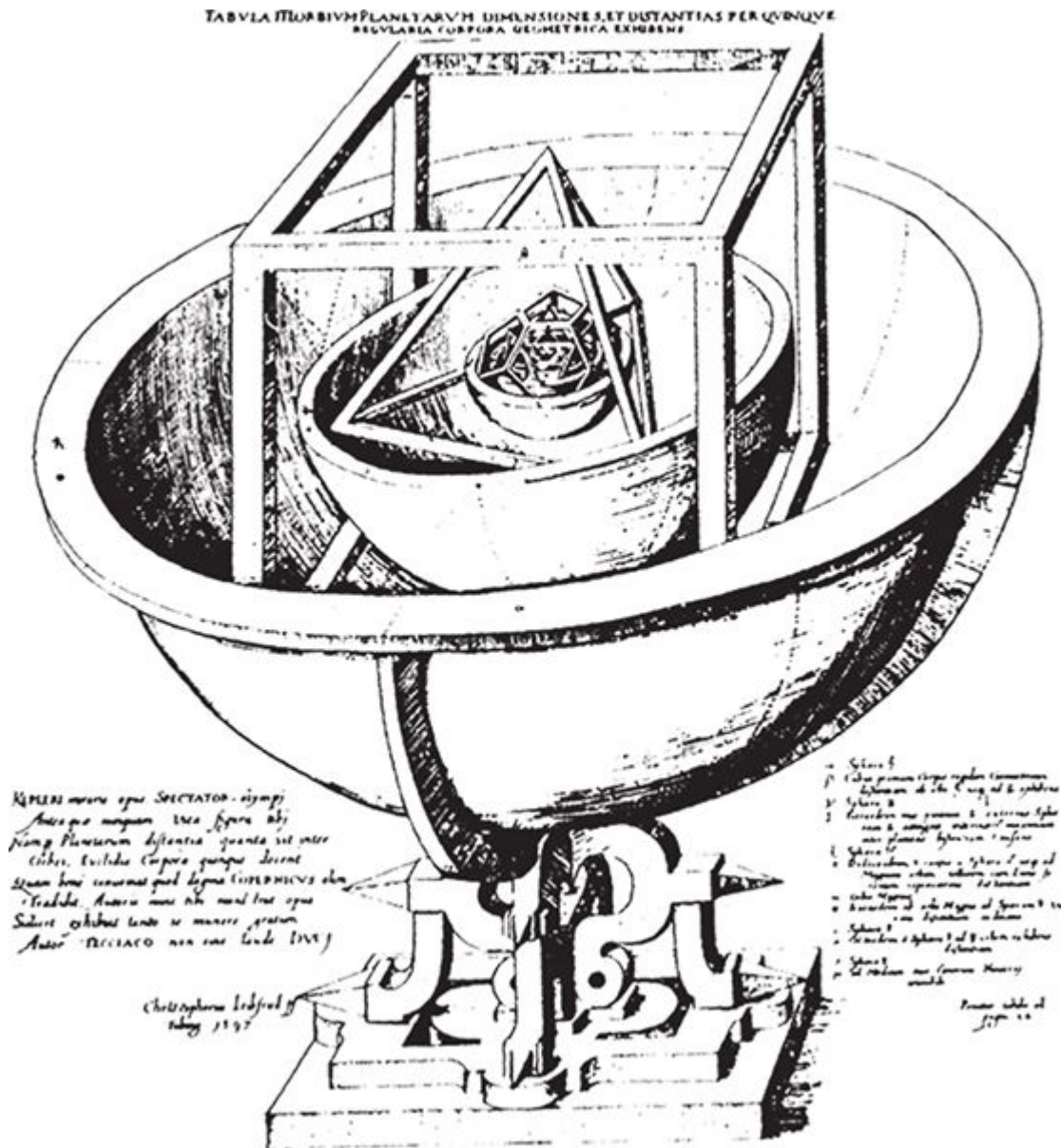
FIGURA 9. Modelo de Kepler para a distância entre as órbitas planetárias, baseado nos cinco poliedros regulares (publicado em 1596).
