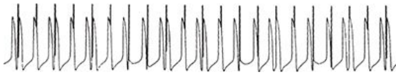
FIGURA 119. O fenômeno Wenckebach: flutuações irregulares do batimento cardíaco. Observe a ausência de padrão regular no espaçamento entre os picos largos e estreitos.
