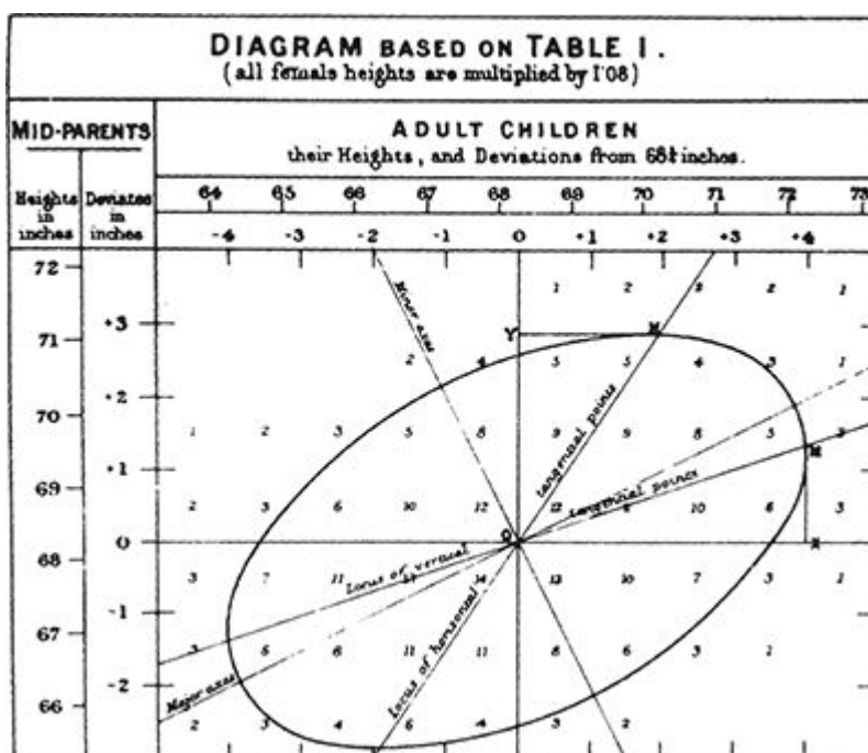
FIGURA 19. O diagrama de Francis Galton da relação entre as alturas dos filhos e as de seus pais, mostrando um padrão de elipses concêntricas.
