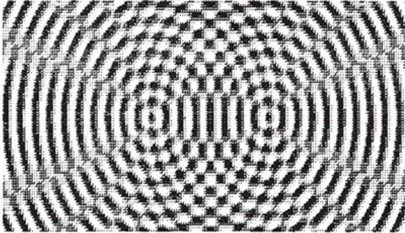
FIGURA 30. Franjas de interferência formadas pela superposição de duas ondas.
