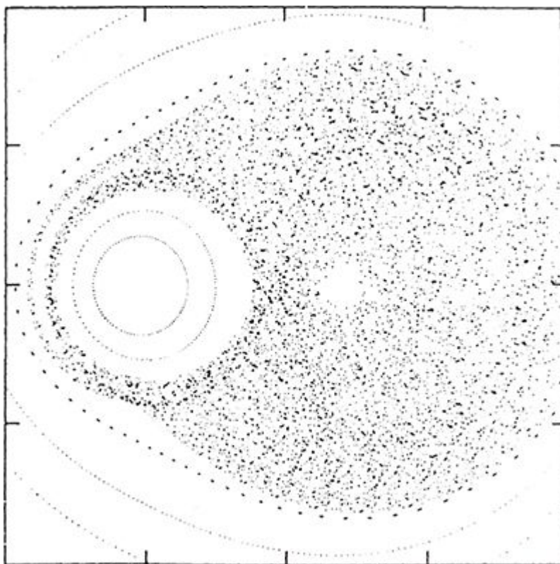
FIGURA 111. A seção de Poincaré para um asteroide em ressonância 3:1 com Júpiter tem duas faixas caóticas distintas, explicando os picos de excentricidade.
