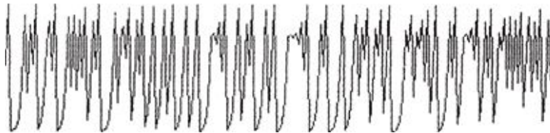
FIGURA 7. A iteração de 2x^2 - 1 conduz ao caos.
