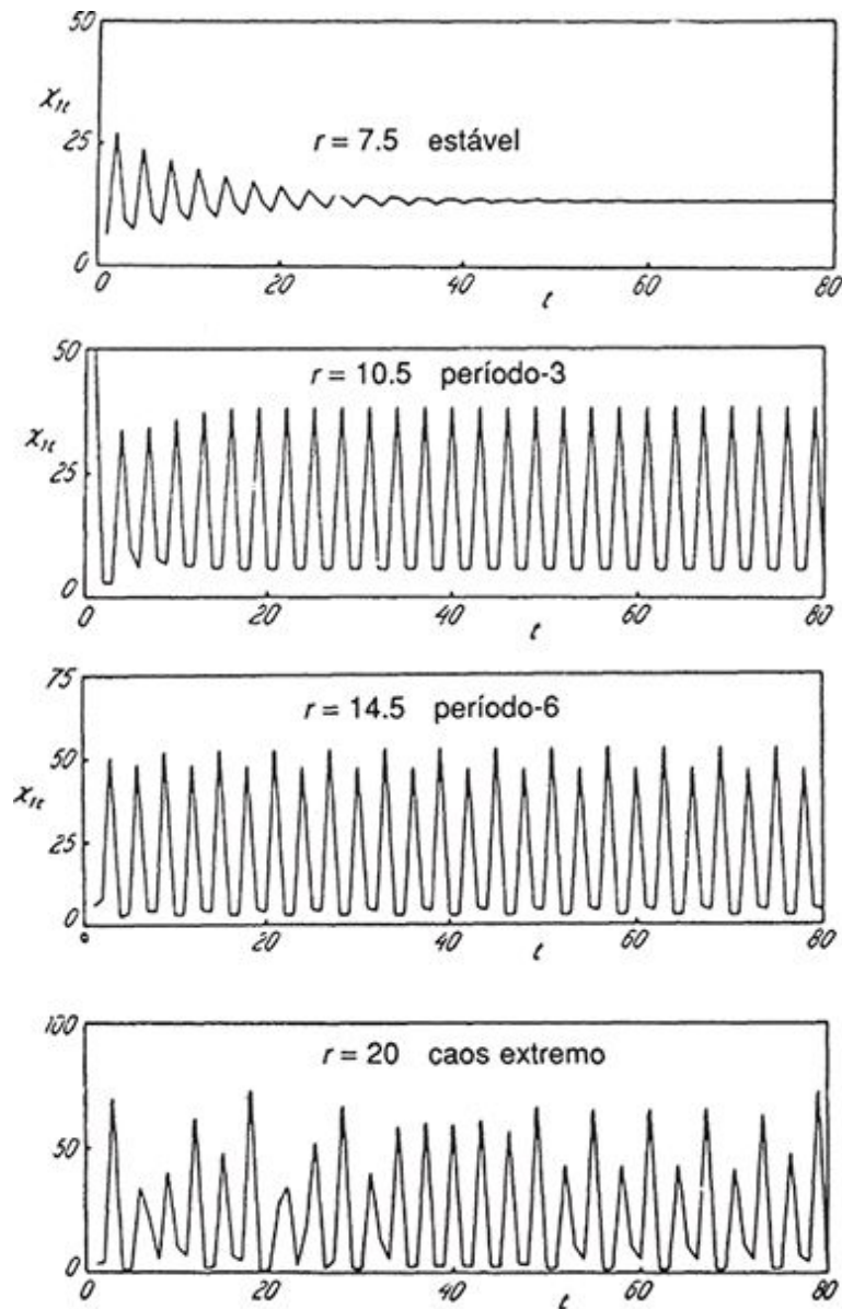
FIGURA 116. Períodos múltiplos e caos no modelo de ciclos populacionais de George Oster.
