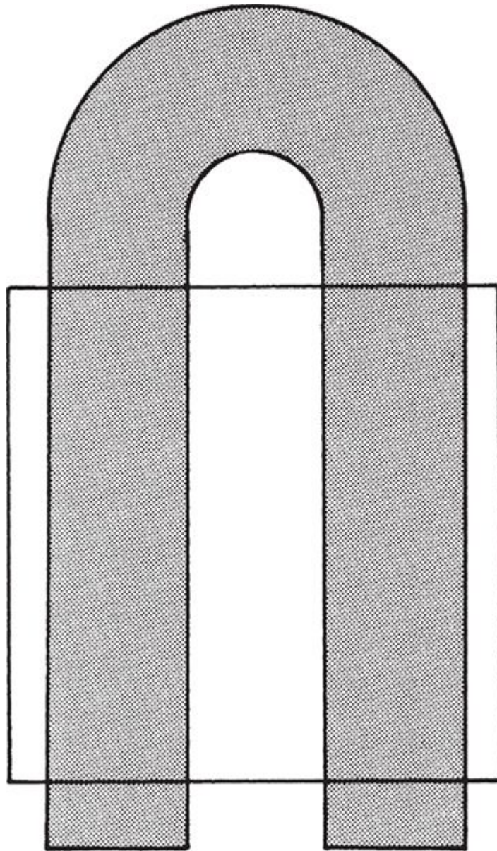
FIGURA 58. O mapeamento da ferradura, de Smale, simula um dobramento caótico. Um quadrado é esticado, dobrado e reintroduzido em si mesmo. Quando iterado, o mapeamento produz uma intrincada estrutura de múltiplas camadas.
