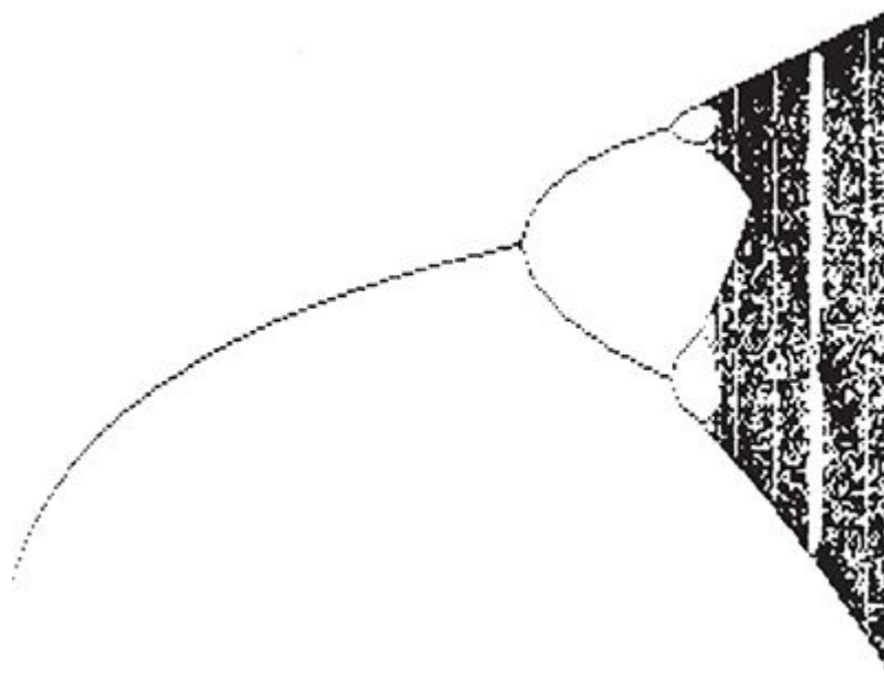
FIGURA 83. A figueira: uma cascata duplicadora de período no mapeamento trigonométrico (compare com a figura 65).
