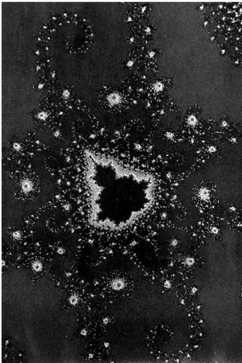
FIGURA 103. ... e revela um sub-boneco de pão de mel, perfeito em todos os detalhes! (Reprodução autorizada de H.-O. Peitgen e P.H. Richter: The Beauty of Fractals , 1986. © 1986 Springer-Verlag Berlim – Heidelberg.)
