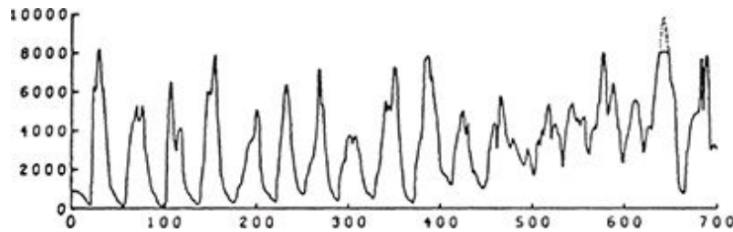
FIGURA 113. Flutuações numa população de moscas-varejeiras. A escala de tempo horizontal é medida em dias.
