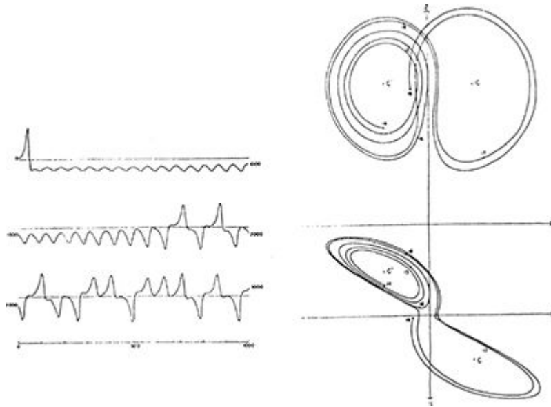
FIGURA 54. Gráficos feitos por Lorenz, representando 3.000 passos numericamente computados em suas equações para a convecção: (à esquerda) as oscilações crescem e se tornam caóticas; (à direita) duas visões do movimento no espaço de fase. (American Meteorological Society, Journal of the Atmospheric Sciences , vol. 20 [Edward N. Lorenz].)
