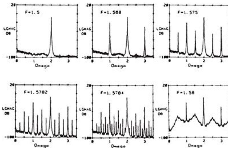
FIGURA 87. Evidência experimental de uma figueira na convecção. Cada novo conjunto de picos ocorre a intervalos que são a metade dos anteriores, indicando a duplicação de período. Pode-se ver uma sequência de quatro duplicações de períodos, seguida por caos.
