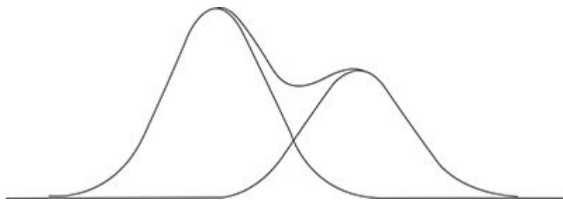
FIGURA 18. A superposição de duas distribuições normais pode produzir uma curva com dois picos.
