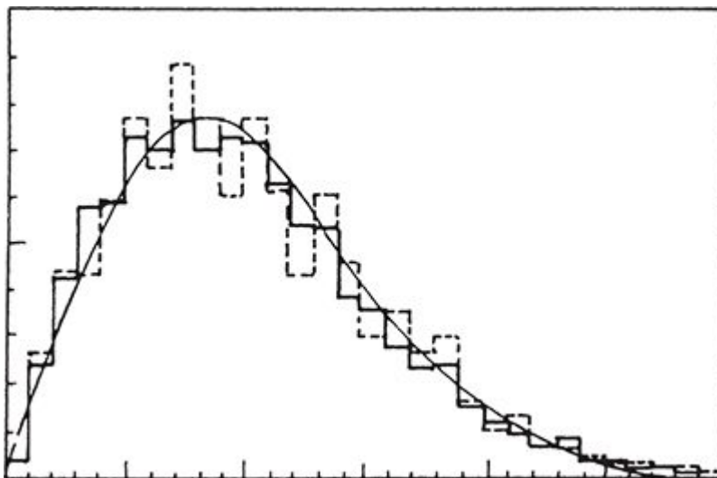
FIGURA 123. Quando os dois sistemas da figura 122 são quantizados, as lacunas entre os níveis de energia de suas funções de onda têm diferentes propriedades estatísticas. A figura mostra os desvios em relação à média teórica (linha curva) para o bilhar circular (linha pontilhada) e o estádio (linha sólida).
