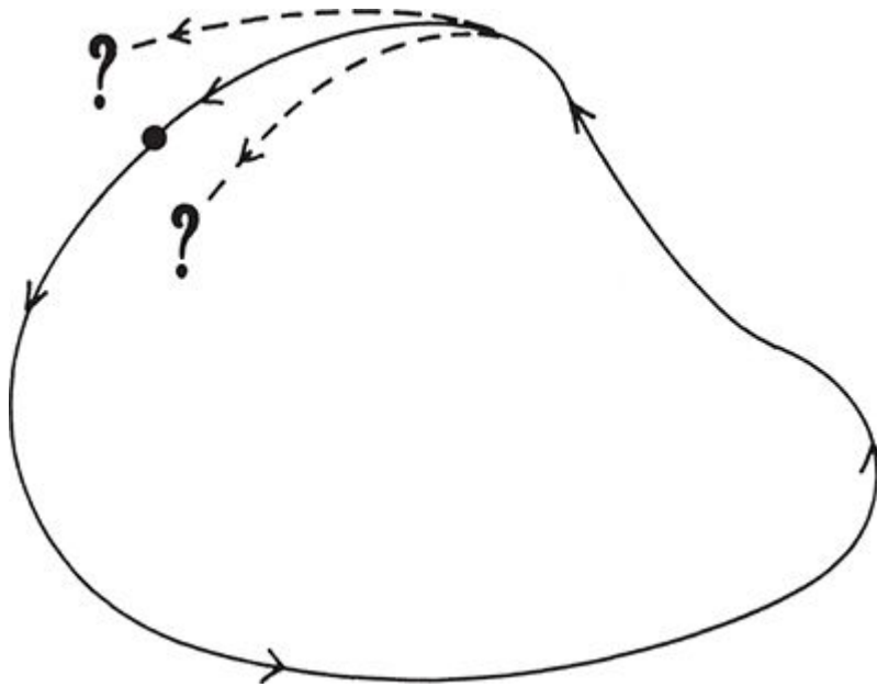
FIGURA 24. Se um ponto em espaço de fase traça um ciclo fechado, ele repetirá periodicamente o mesmo movimento para sempre.
