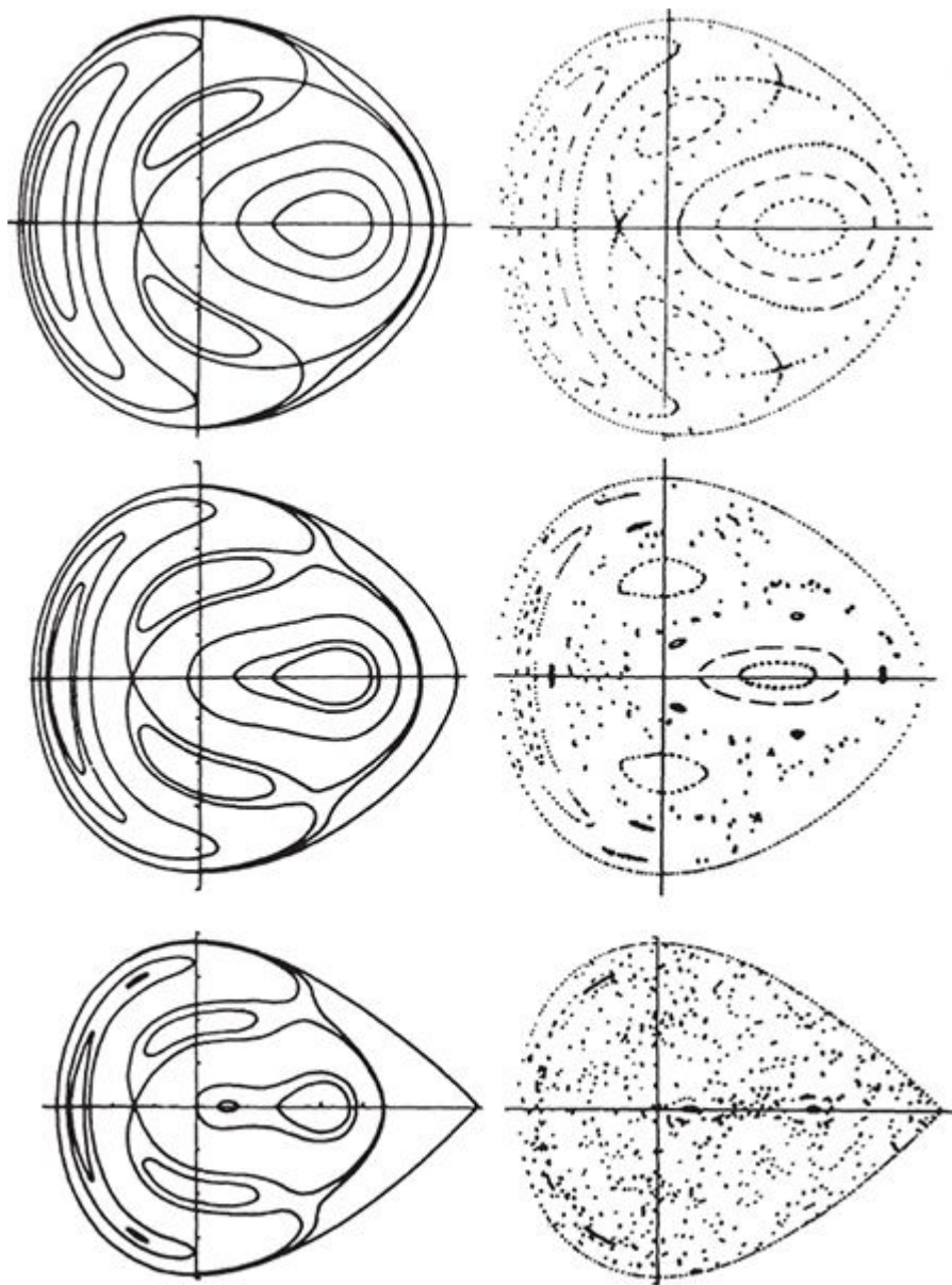
FIGURA 59. O problema dos três corpos, numa aproximação de Hénon e Heiles: (à esquerda) trajetórias computadas por aproximações de séries clássicas são sempre regulares na forma; (à
