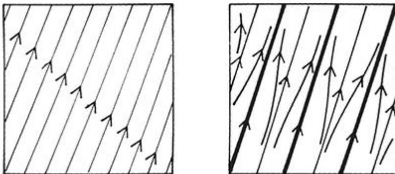
FIGURA 71. Engate de frequências: (à esquerda) duas oscilações periódicas independentes combinadas por sua superposição; (à direita) o fluxo se fragmenta para formar um ciclo periódico estável (linha mais grossa) e um ciclo periódico instável. Para efeito de maior clareza, o toro em que o movimento ocorre foi cortado e aberto de modo a formar um quadrado.
