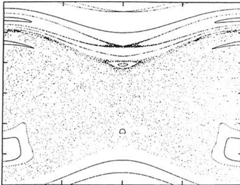
FIGURA 106. Uma seção de Poincaré para Hipérion. A região pontilhada indica movimento caótico: todos os pontos correspondem a uma única trajetória. As voltas fechadas indicam regiões de movimento regular quase-periódico.
