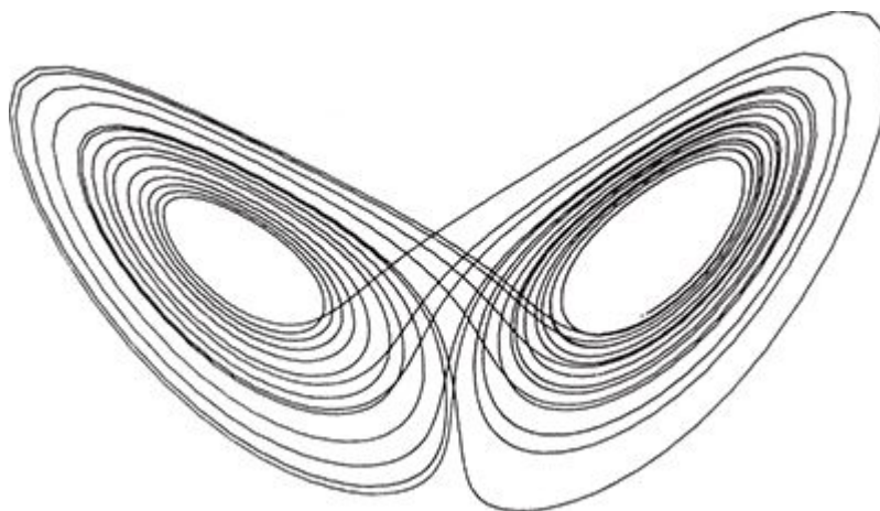
FIGURA 55. O atrator de Lorenz: trajetórias giram, de maneira aparentemente aleatória, em torno dos dois lobos.
