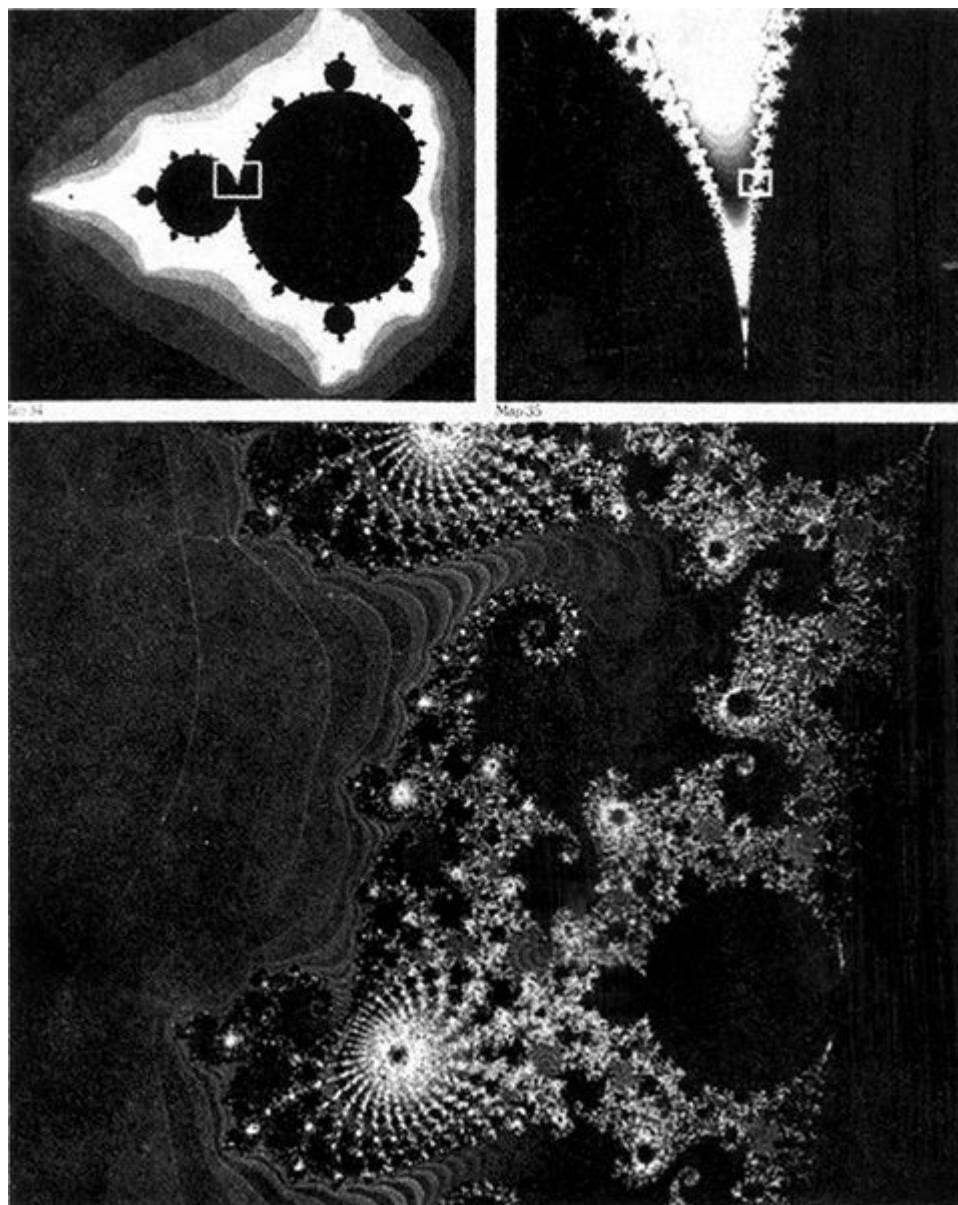
FIGURA 101. Um zoom no boneco de pão de mel... (Reprodução autorizada de H.-O. Peitgen e P.H. Richter: The Beauty of Fractals , 1986. © 1986 Springer-Verlag Berlin – Heidelberg.)
