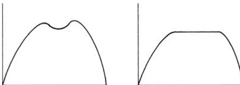
FIGURA 85. Mapeamentos com múltiplas corcovas ou uma corcova achatada levam a diferentes feigenvalores.
