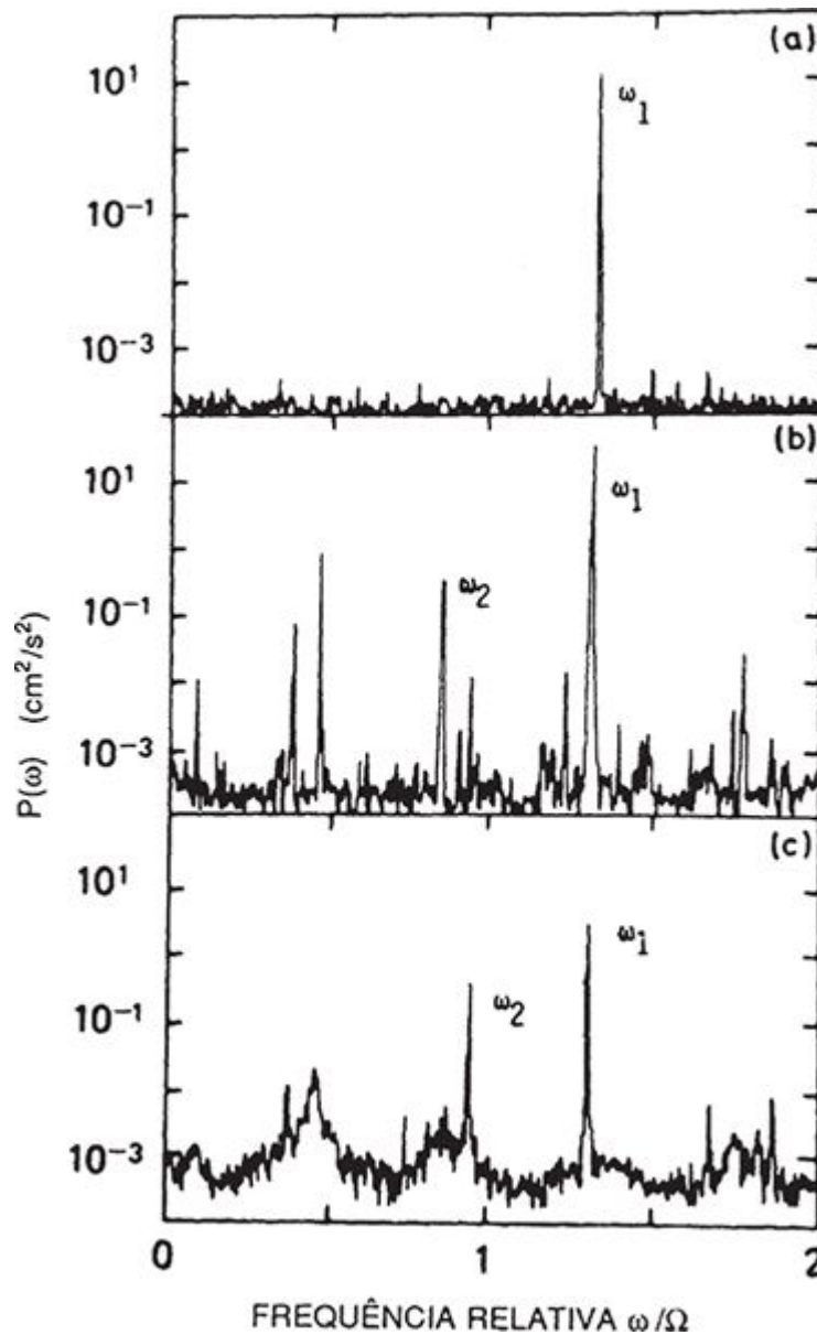
FIGURA 75. Espectro de potência para o sistema de Taylor-Couette. Inicialmente, só uma frequência \omega_1 é observada (oscilação periódica). Depois uma segunda frequência \omega_2 aparece (juntamente com outras pontas que representam combinações de \omega_1 e \omega_2 ). Por fim, bandas largas de caos podem ser vistas. (Reproduzido com a permissão de John Wiley & Sons Ltd.)
