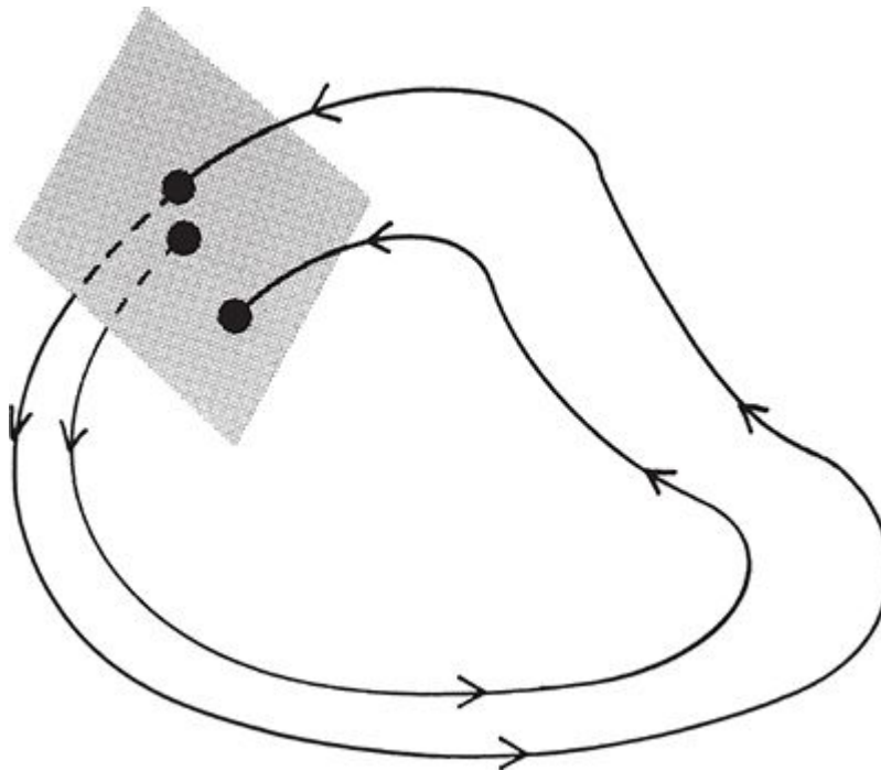
FIGURA 25. Detecção de um movimento periódico por meio da seção de Poincaré. Para haver periodicidade, a curva deve retornar à seção exatamente no ponto de partida.
