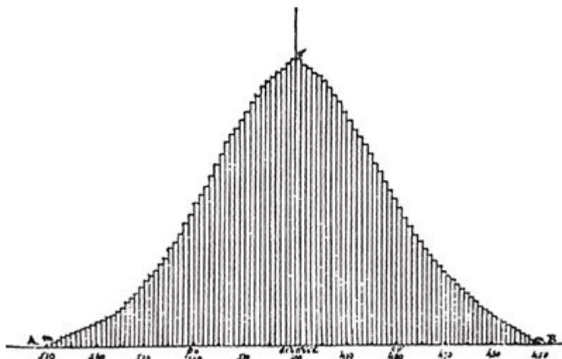
FIGURA 16. Aproximação binomial a uma distribuição normal (Quetelet, 1846).
