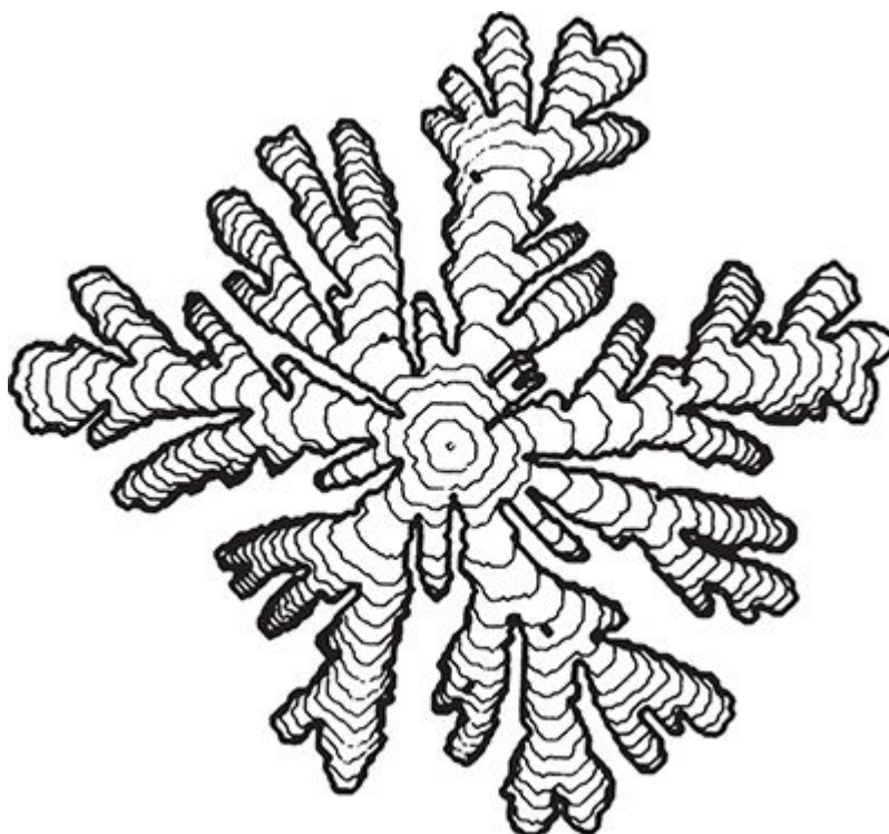
FIGURA 93. Dedos viscosos de óleo bombeado na água. (Reprodução autorizada de Nature , vol. 321, p.668, © Macmillan Magazines Ltd.)
