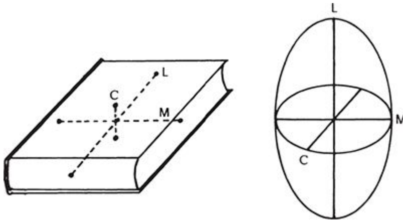
FIGURA 105. Um livro e seu elipsoide inercial. Observe que o eixo mais curto (C) do livro corresponde ao eixo mais longo (L) do elipsoide, e vice-versa, e que os dois eixos médios (M) se correspondem.
