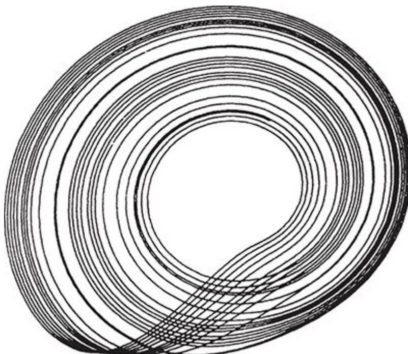
FIGURA 79. O atrator de Rössler.
