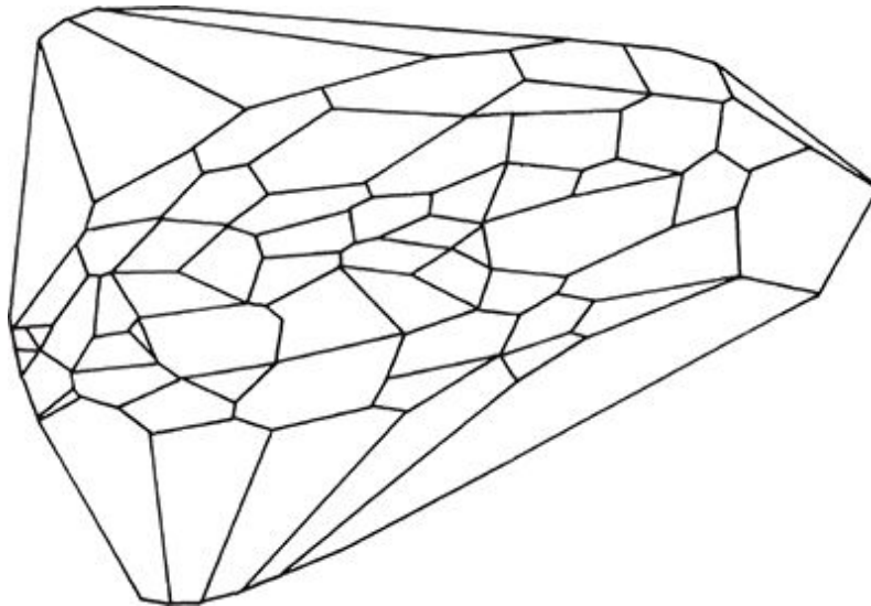
FIGURA 35. Projeção tridimensional de um poliedro multidimensional que ocorre numa aplicação do algoritmo de Karmarkar. (Reproduzido com a permissão de AT&T Bell Laboratories Record, © 1986 AT&T.)
