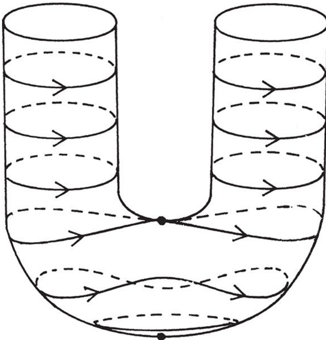
FIGURA 32. Representação geométrica da conservação da energia. Se o espaço de fase cilíndrico de pêndulo for encurvado, na forma de um tubo em U, as trajetórias permanecem em alturas constantes.
