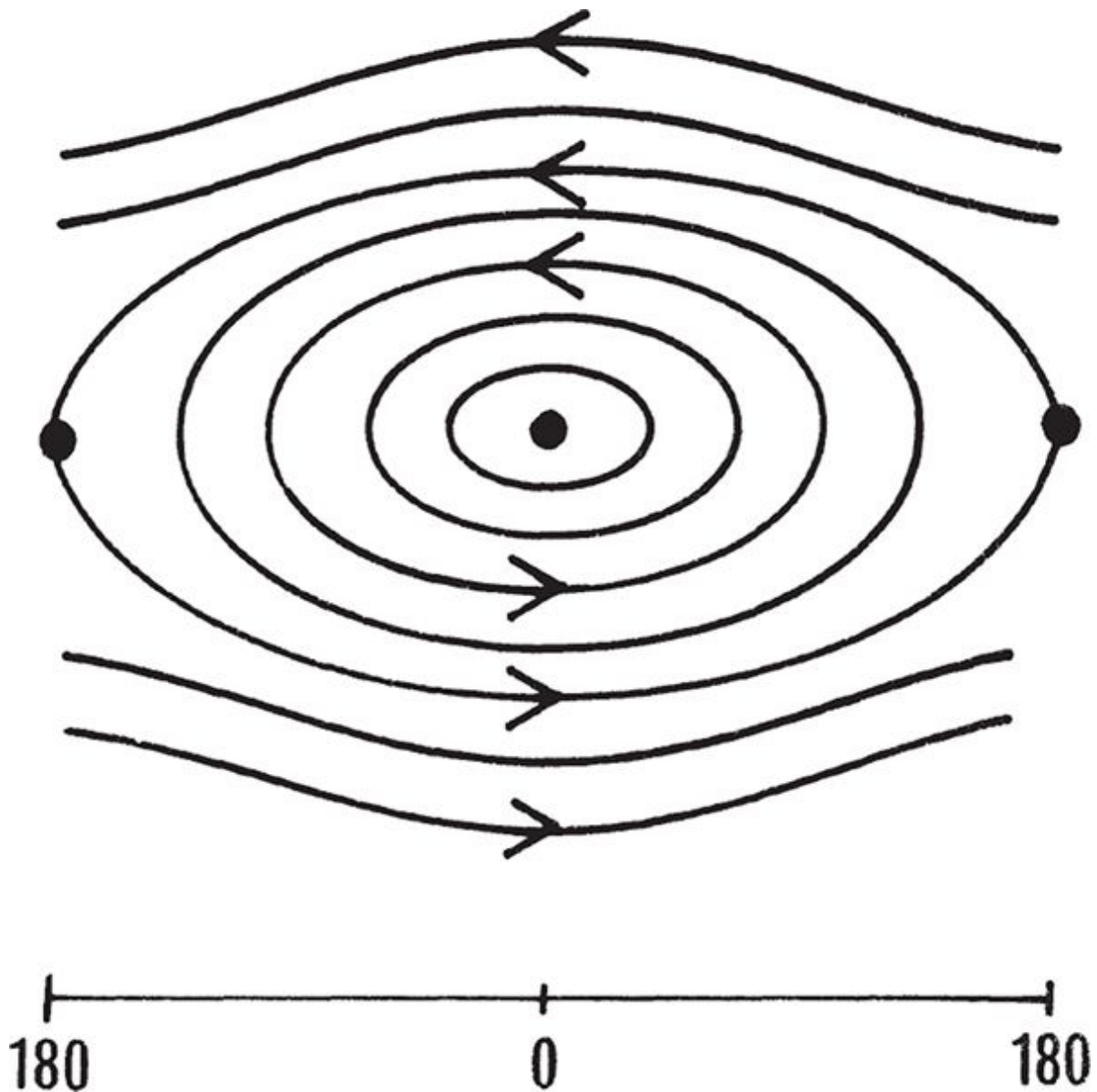
FIGURA 29. Retrato de fase de um pêndulo não linear “genuíno”.
