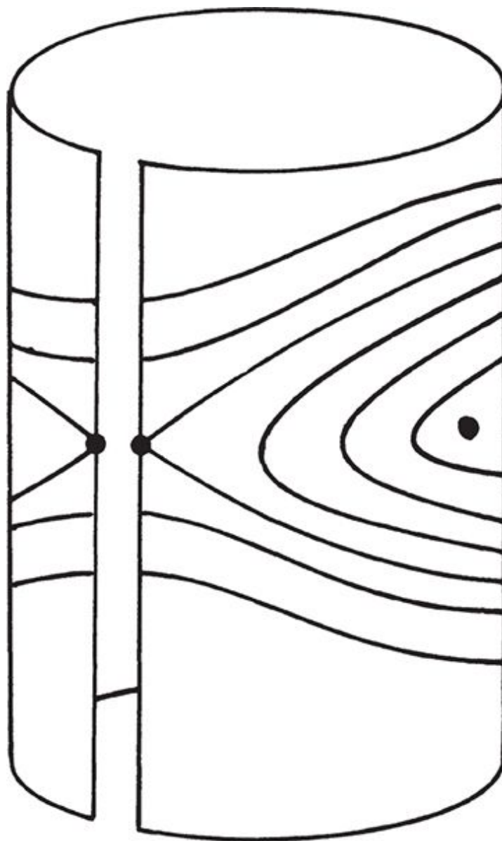
FIGURA 31. Enrolando-se o plano de fase de um pêndulo, de modo a formar um cilindro, obtém-se uma representação mais aproximada de sua posição, que é um ângulo.
