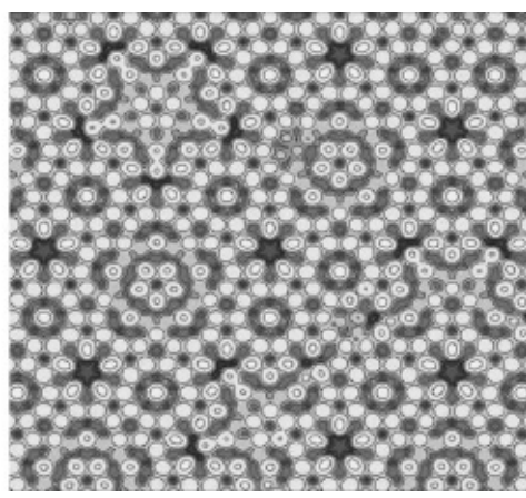
FIG 41 Esquerda : Um dos dois padrões de quase-cristais com exata simetria quántupla. Direita : Modelo atômico do quasecristal icosaédrico alumínio-paládio-manganês.
