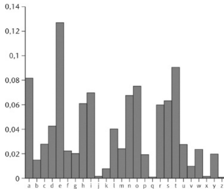
FIG 157 Gráfico da frequência de uma dada letra num texto típico em inglês.
