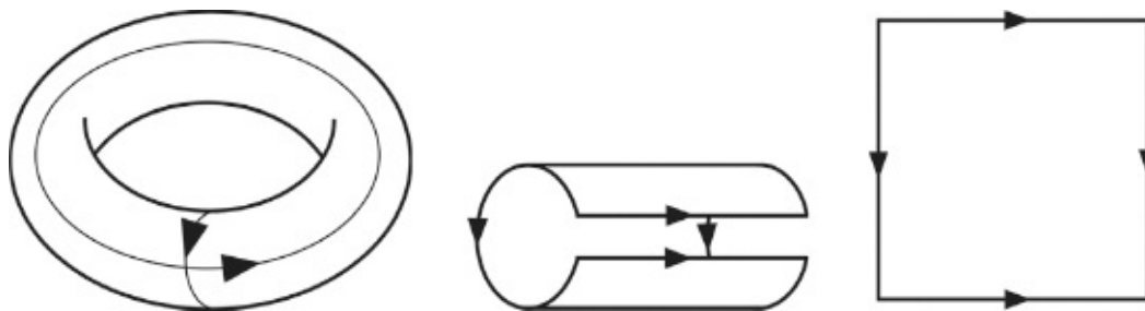
FIG 46 Aplainando um toro de modo a formar um quadrado.
