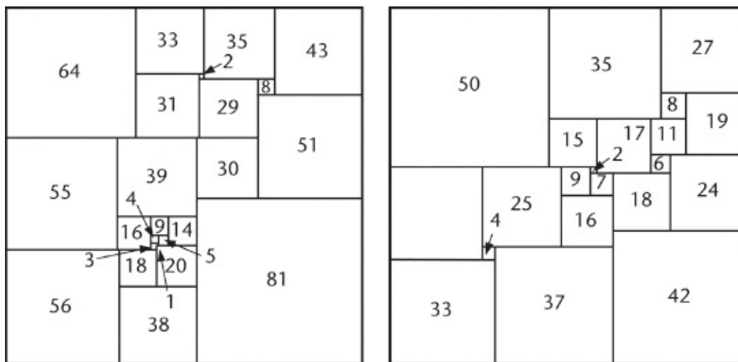
FIG 57 Esquerda : Quadrado quadriculado de Willcocks com 24 ladrilhos. Direita : Quadrado de Duijvestijn com 21 ladrilhos.
