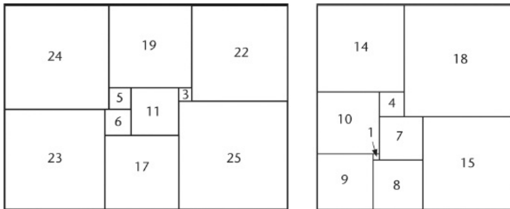
FIG 56 Esquerda : Primeiro retângulo quadriculado de Morón. Direita : Seu aperfeiçoamento para nove ladrilhos.
