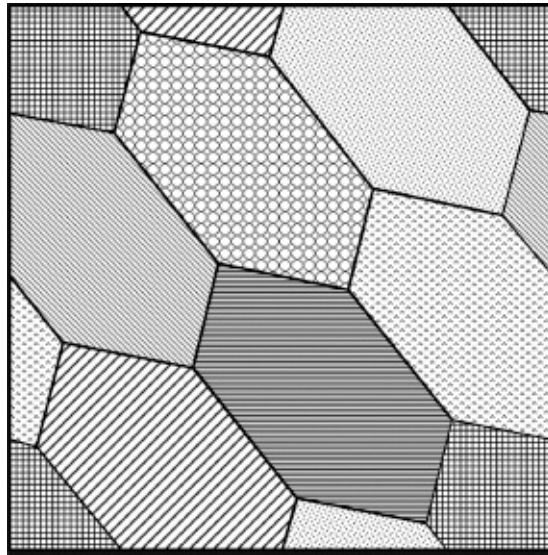
FIG 47 Um mapa sobre um toro necessitando de sete cores.
