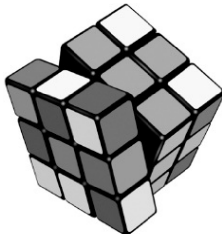
FIG 171 Cubo de Rubik.
