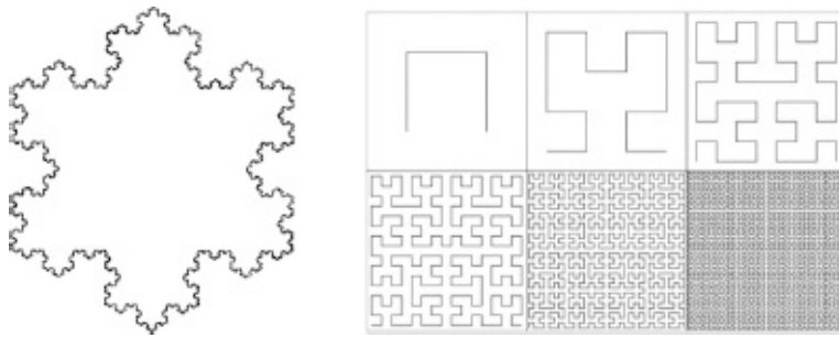
FIG 109 Esquerda : Curva do floco de neve. Direita : Estágios sucessivos da construção da curva de preenchimento de espaço de Hilbert.
