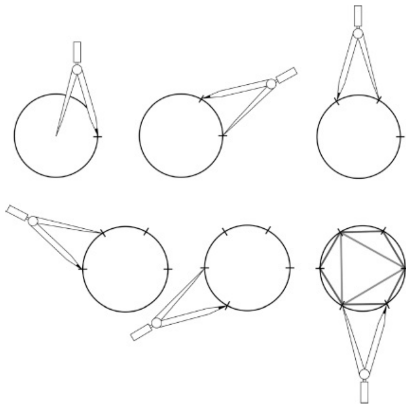
FIG 142 Desenhe um círculo e marque um ponto nele. A partir desse ponto, vá marcando outros pontos sucessivos mantendo a mesma abertura do compasso (o último ponto coincidirá com o inicial). Isso produz os seis vértices de um hexágono regular. Tomando cada segundo vértice teremos um triângulo equilátero.
