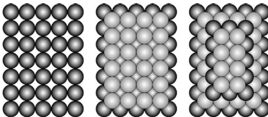
FIG 120 Reticulado CFC. Esquerda: a primeira camada. Centro: primeiras duas camadas. Direita: Primeiras quatro camadas.
