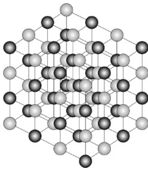
FIG 40 Reticulado cristalino do sal. Esferas escuras: átomos de sódio. Esferas claras: átomos de cloro.
