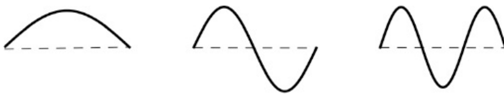
FIG 126 Instantâneos de modos 1, 2, 3 de uma corda vibratória. Em cada caso a corda vibra para cima e para baixo, e sua amplitude varia senoidalmente com o tempo. Quanto mais ondas houver, mais rápida a vibração.
