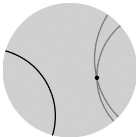
FIG 164 Modelo do disco de Poincaré do plano hiperbólico (sombreado). As duas retas de cor cinza são paralelas à reta preta e passam pelo mesmo ponto.
