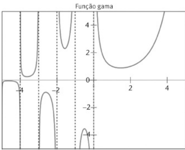
FIG 170 Gráfico de \Gamma(x) para x real.
