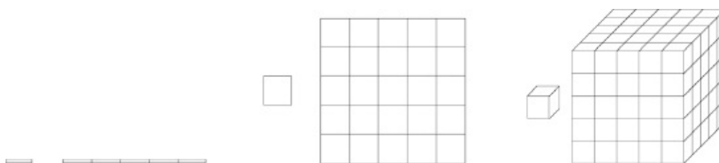
FIG 114 Efeito de escala em “cubos” em 1, 2 e 3 dimensões.
