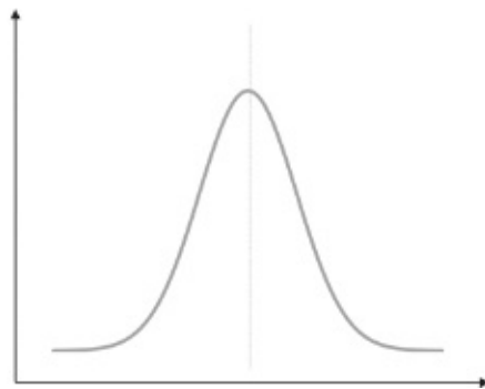
FIG 100 A curva do sino.
