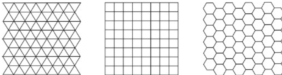
FIG 21 Três modos de ladrilhar o plano: triângulos equiláteros, quadrados e hexágonos.
