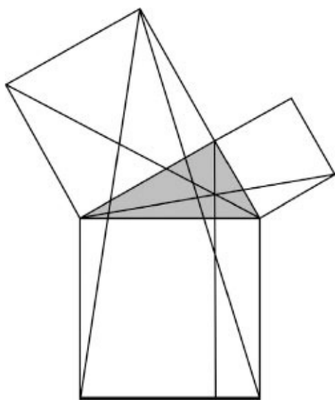
FIG 33 As calças de Pitágoras.
