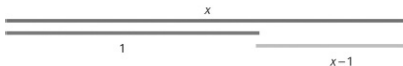
FIG 103 Divisão em extrema e média razão: a razão do segmento cinza-escuro (1) para o segmento cinza-claro ( x - 1 ) é igual à razão do segmento preto ( x ) para o segmento cinza-escuro (1).
