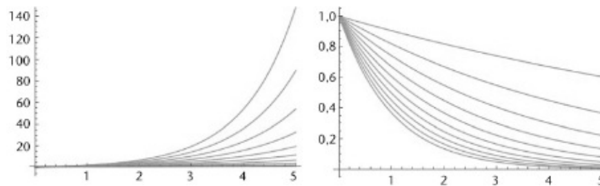
FIG 107 Esquerda: Crescimento exponencial e^{kt} para k = 0,1; 0,2;\dots;1 . Direita: Decréscimo exponencial e^{-kt} para k = 0,1; 0,2;\dots;1 .
