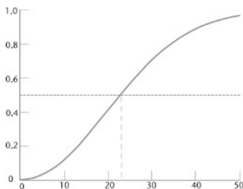
FIG 154 Como P(k) depende de k .
