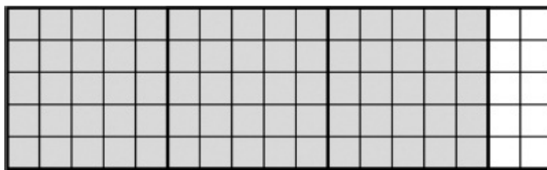
FIG 92 Recorte três quadrados 5 \times 5 .
