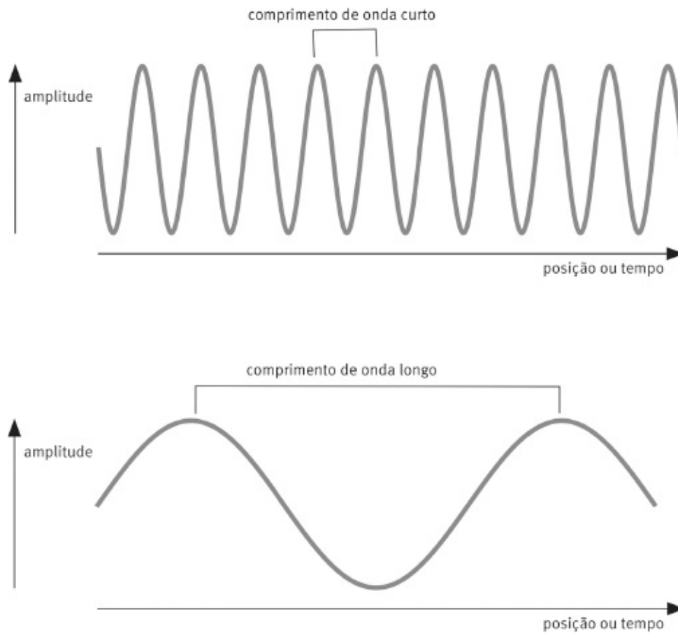
FIG 122 Comprimento de onda.
