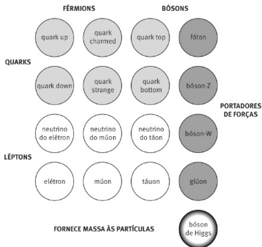
FIG 131 As dezessete partículas fundamentais.
